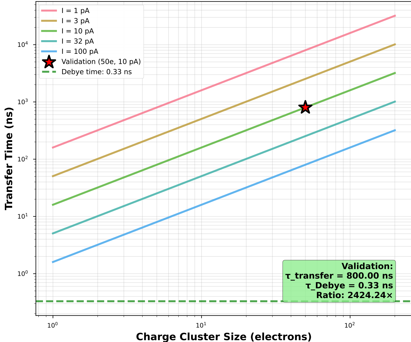
(D) Classical vs Quantum Charge Transfer
