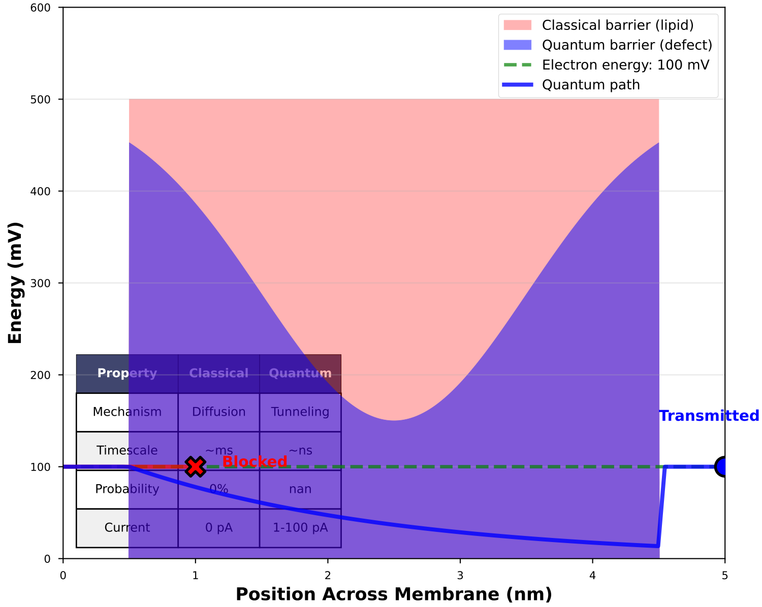
(D) Classical vs Quantum Charge Transfer
