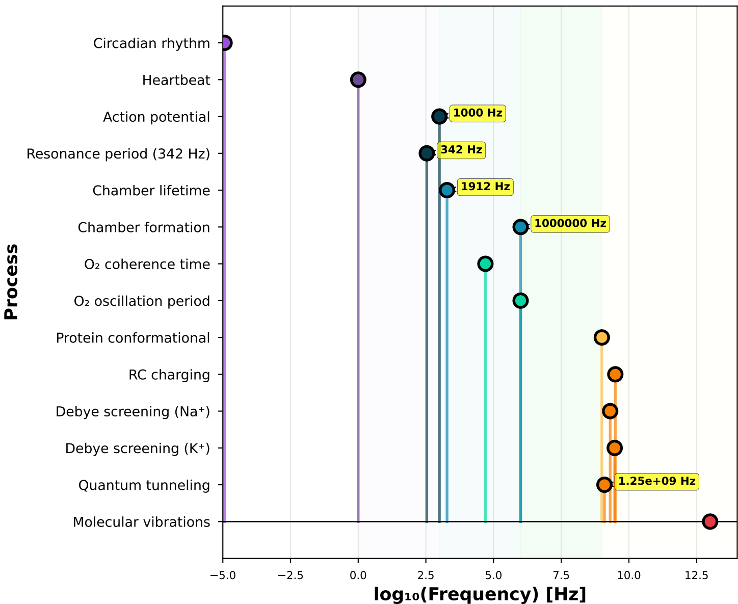
(D) Physiological Oscillations: Multi-Scale Coherence
