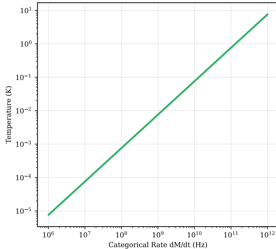
T = \hbar(dM/dt)/k_B
