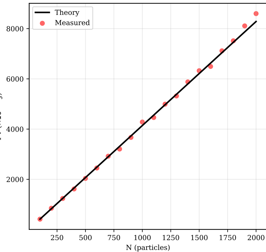
PV = NkT
