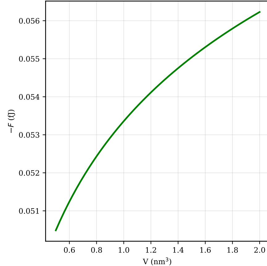
F = -k_B T \ln Z
