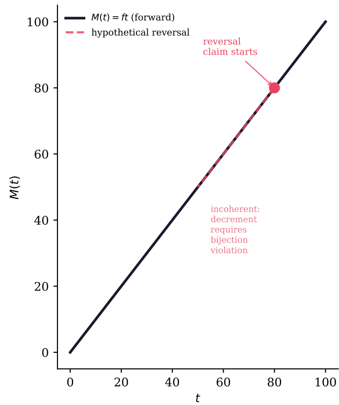
Monotone M(t) : No Reversal
