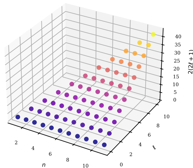
Sublevel Degeneracy
