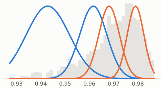
L25_cos
