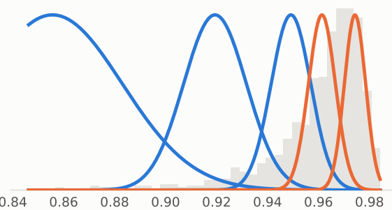
L27_cos
