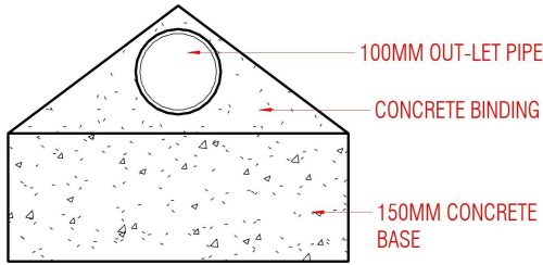
SECTION 3 1 : 10
