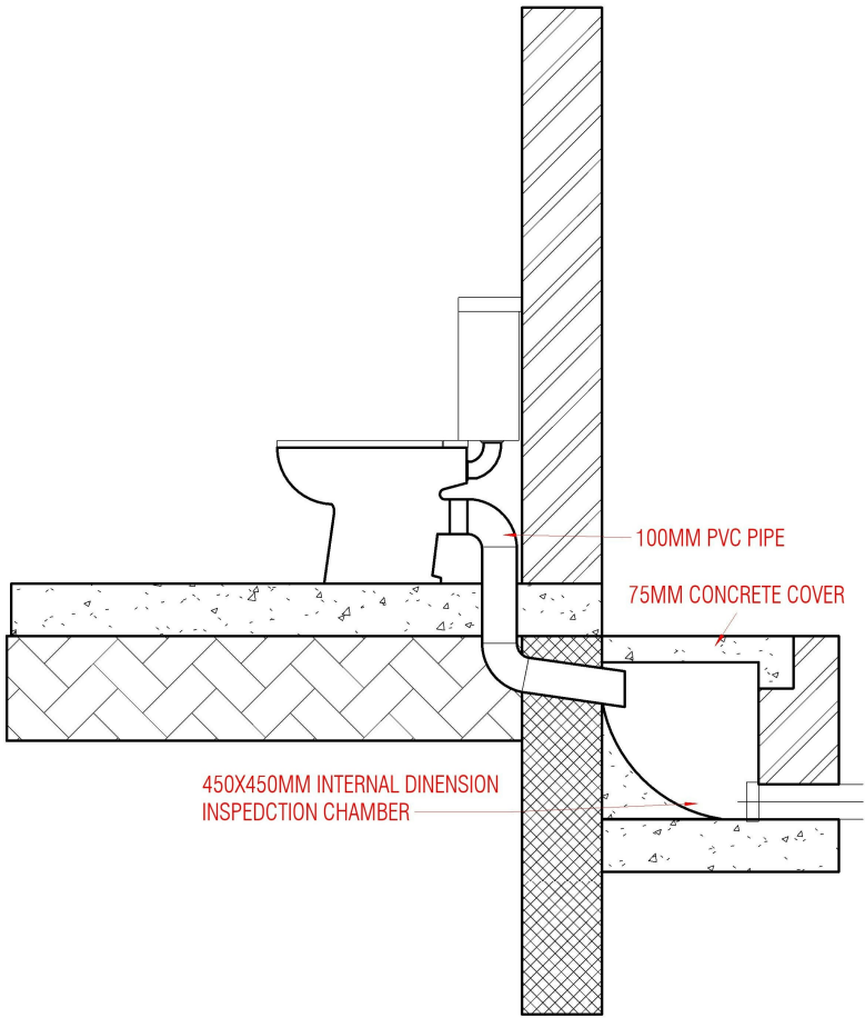
WC DETAIL 1 : 25
