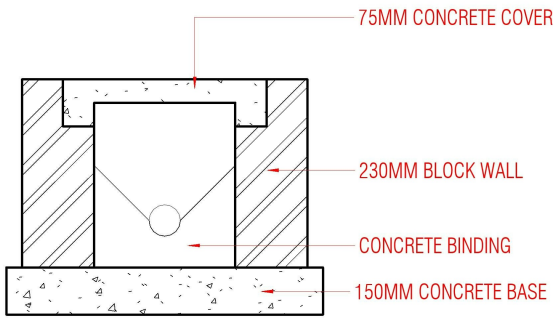
SECTION 2 1 : 25
