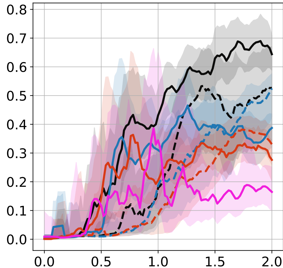
ZIGZAG
