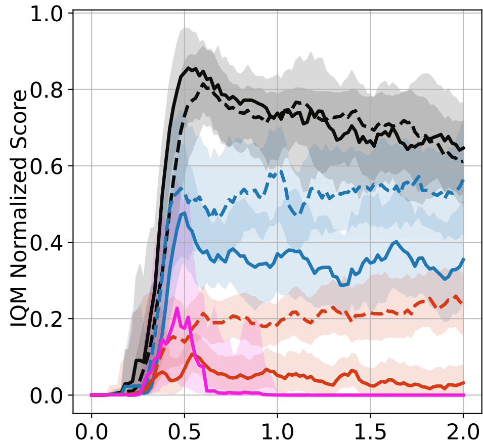
CLIFFWALKING
