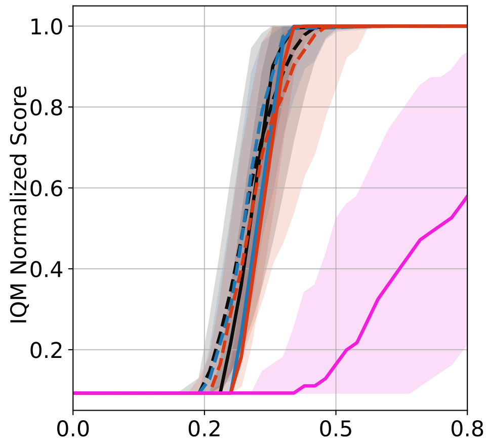
CLIFFWALKING
