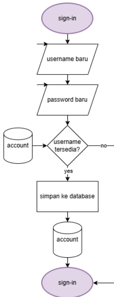
Gambar 2.3 Fungsi Registrasi
