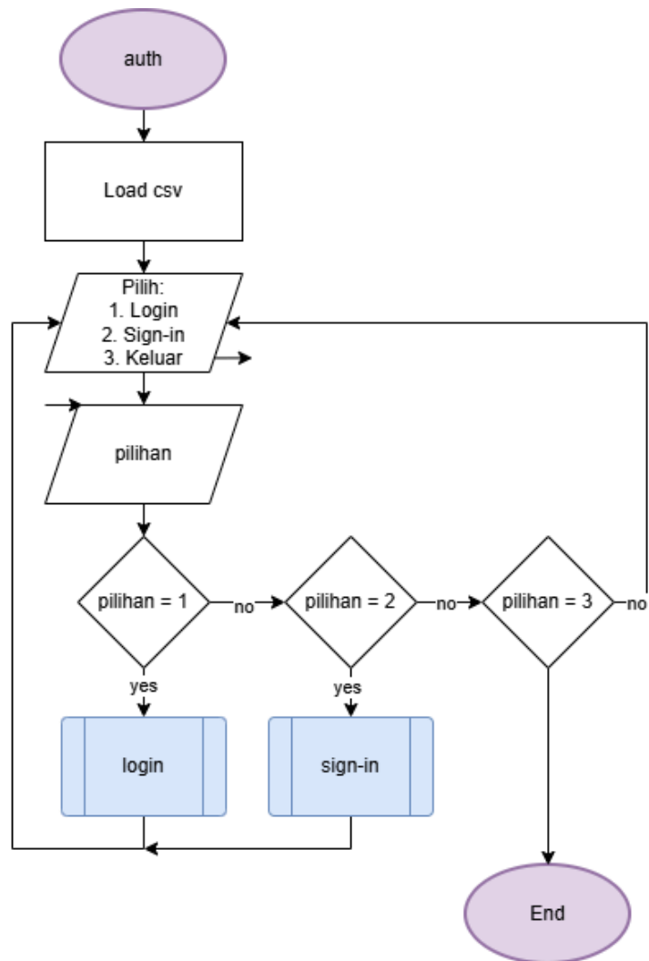
Gambar 2.1 Fungsi Autentikasi
