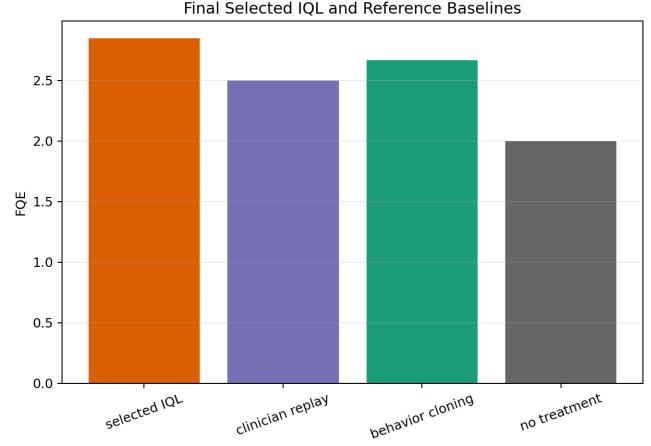
Şekil 2. Final seçili IQL politikası ve referans başlangı çizgisi gösterimi (baseline display). Seçili IQL deęeri gerçek Aşama 2 deęerlendirmesinden, referans başlangı çizgisi ubukları (baseline bars) ise rapor ıktısında (artifakt) kullanılan karşılaştırma gösteriminden gelir.
