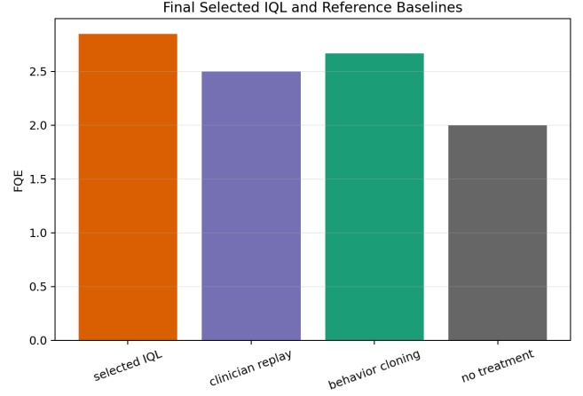
Şekil 2. Final seili IQL politikası ve referans başlangı çizgisi gösterimi (baseline display). Seili IQL deėeri gerçek Aşama 2 deėerlendirmesinden, referans başlangı çizgisi ubukları (baseline bars) ise rapor ıktısında (artifakt) kullanılan karşılaştırma gösteriminden gelir.
