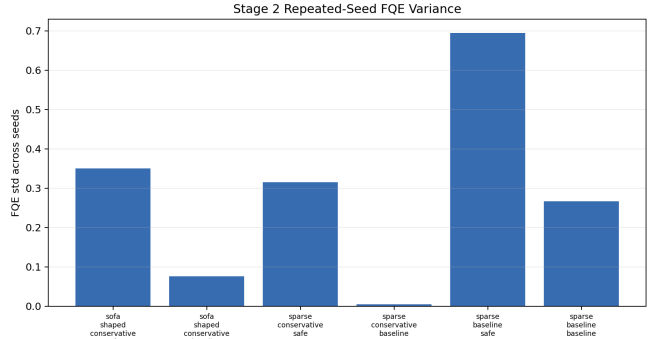
Şekil 3. Aşama 2 finalistleri için tekrarlı-tohum FQE deėişkenliėi. Daha düşük deėer, aynı konfigürasyonun tohumlar arasında daha stabil olduėunu gösterir.
