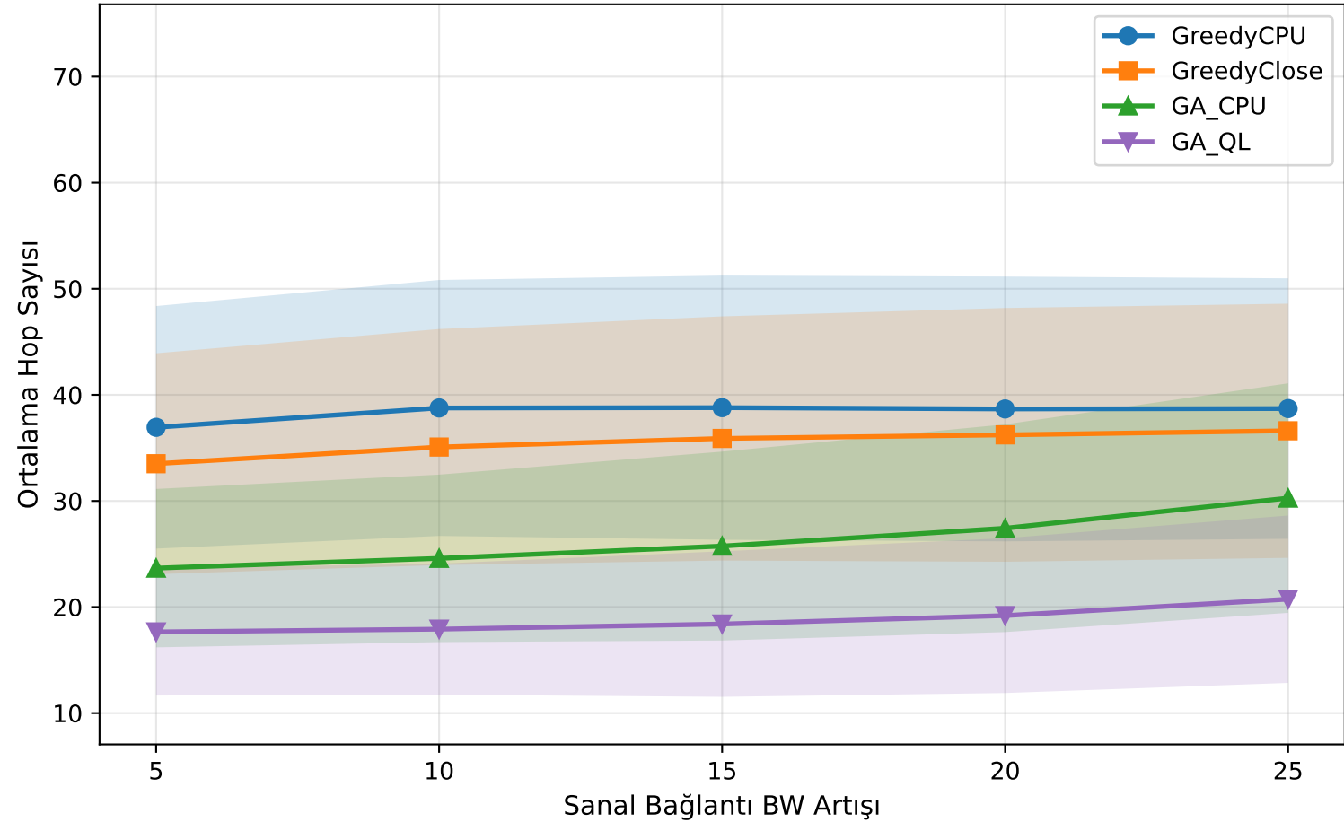
Kabul Edilen İsteklerde Ortalama Hop Sayısı (NSF — VBW Artışı (ISP 6-7-8))
