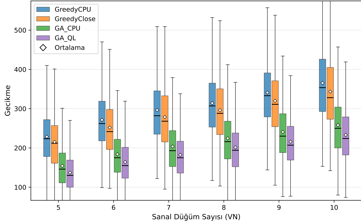
Kabul Edilen İsteklerde Gecikme Dağılımı (NSF — VN Artışı (ISP 6-7-8))
