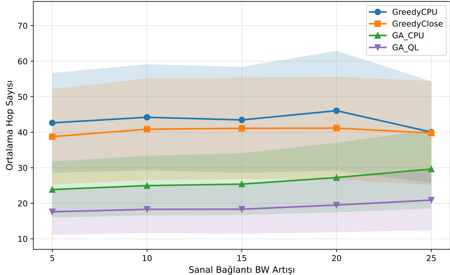
Kabul Edilen İsteklerde Ortalama Hop Sayısı (USnet — VBW Artışı (ISP 6-7-8))
