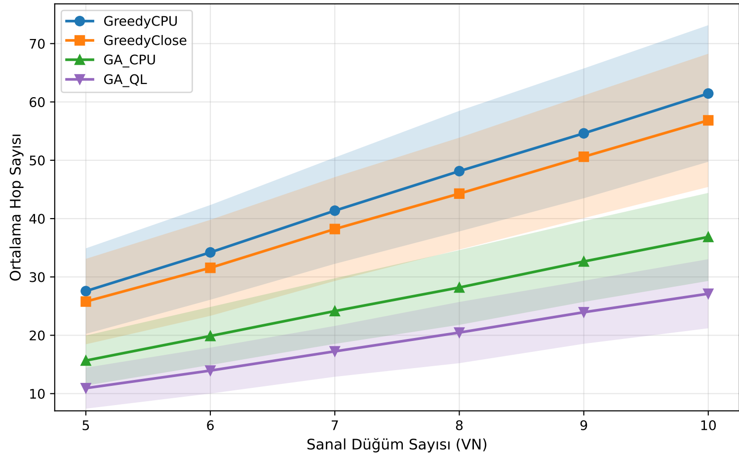
Kabul Edilen İsteklerde Ortalama Hop Sayısı (USnet — VN Artışı (ISP 6-7-8))
