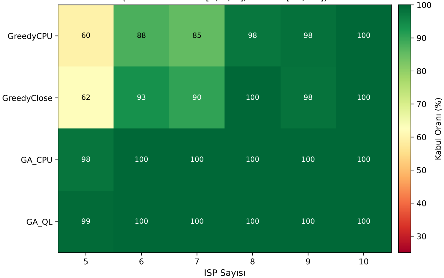
İstek Kabul Oranı (%) (NSF — VNode \in [6, 7, 8] , VBW \in [10, 15] )
