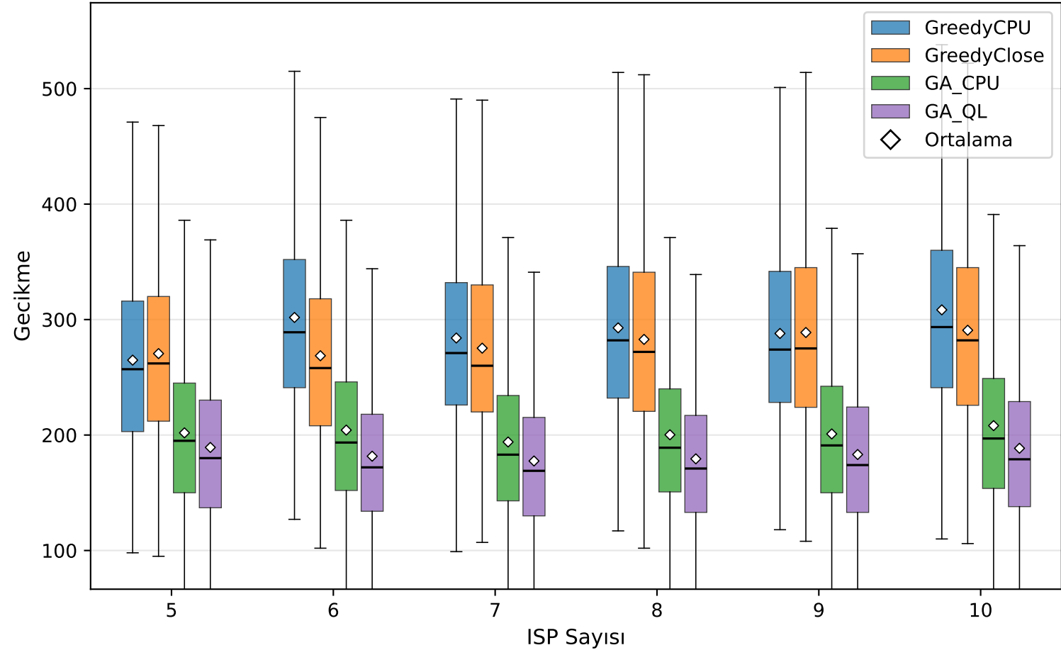
Kabul Edilen İsteklerde Gecikme Dağılımı (NSF — VNode \in [6, 7, 8] , VBW \in [10, 15] )
