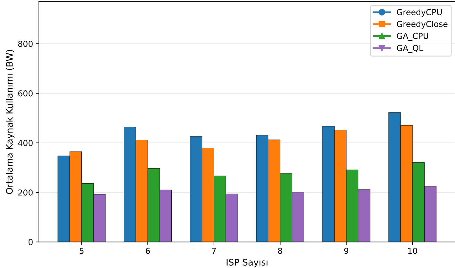
Ortalama Kaynak Kullanımı (BW) (tüm algoritmaların ortak çözdüğü istekler) (NSF — VNode \in [6, 7, 8] , VBW \in [10, 15] )
