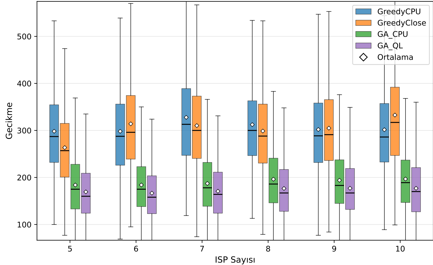
Kabul Edilen İsteklerde Gecikme Dağılımı (USnet — VNode \in [6, 7, 8] , VBW \in [10, 15] )
