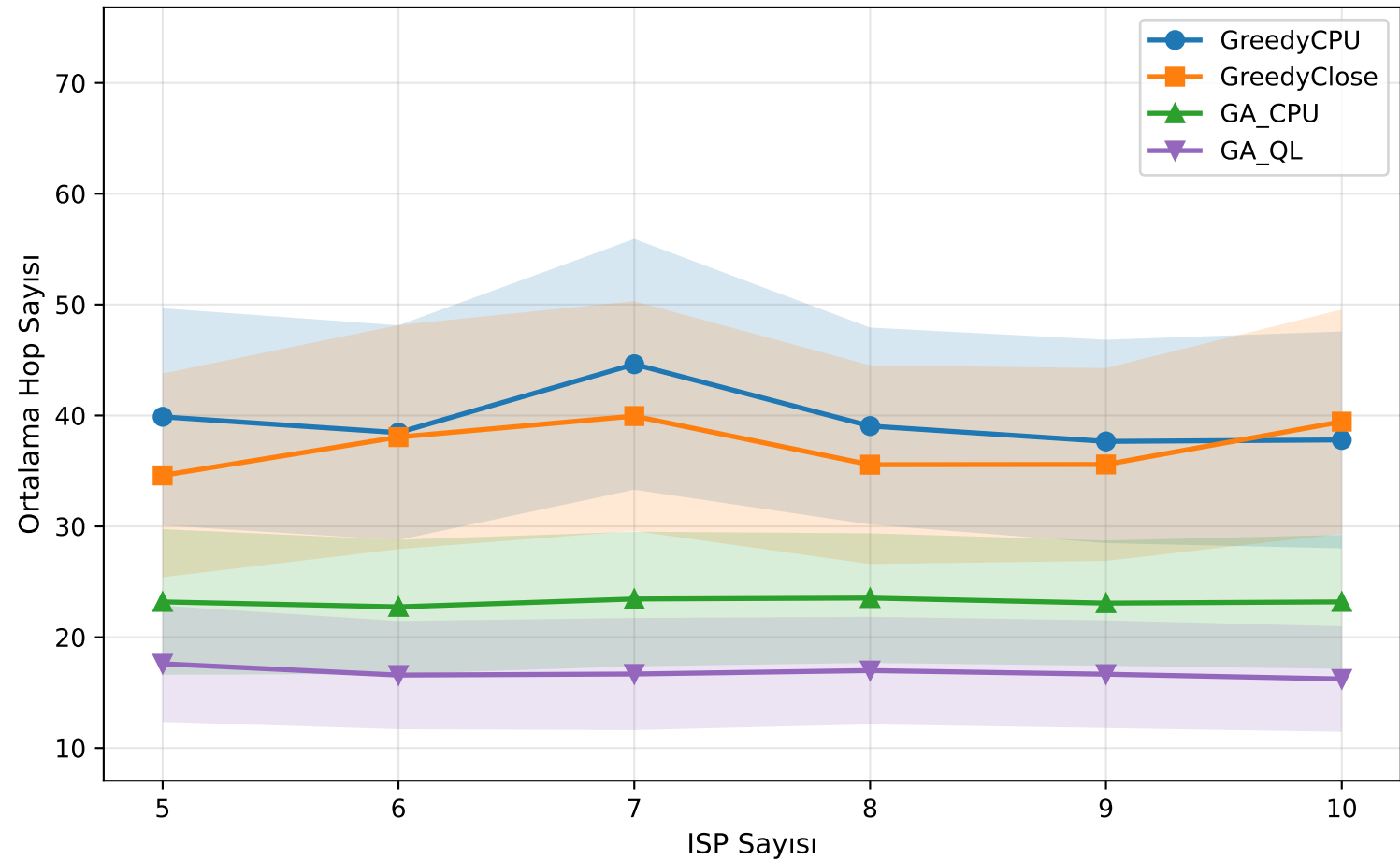
Kabul Edilen İsteklerde Ortalama Hop Sayısı (USnet — VNode \in [6, 7, 8] , VBW \in [10, 15] )
