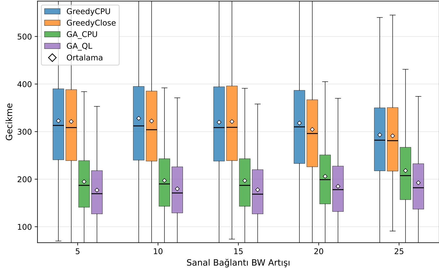
Kabul Edilen İsteklerde Gecikme Dağılımı (USnet — VBW Artışı (ISP 6-7-8))
