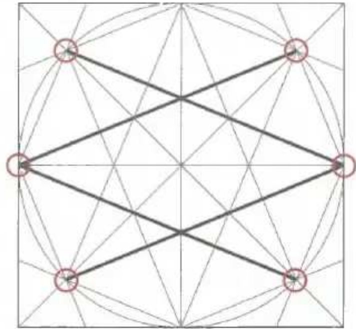
4 Aynı işlemleri takip ederek dört çizgi daha çizin, fakat bu kez karenin dikey kenarlarındaki yuvarlak içine alınmış iki kesişim noktasından başlayın.
