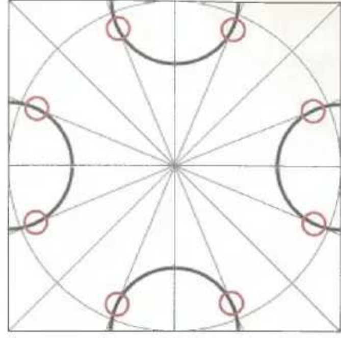
2 Karenin ve dairenin dört kesişim noktasının her birine pergelinizi yerleştirerek, işaretli çizgilerin arasına muntazaman oturacak şekilde dört yay çizin.
