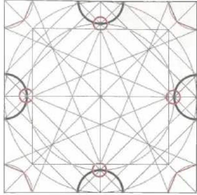
10 7. adımdaki daireye yuvarlak içine alınmış dört noktadan değen dört yay çizin.
