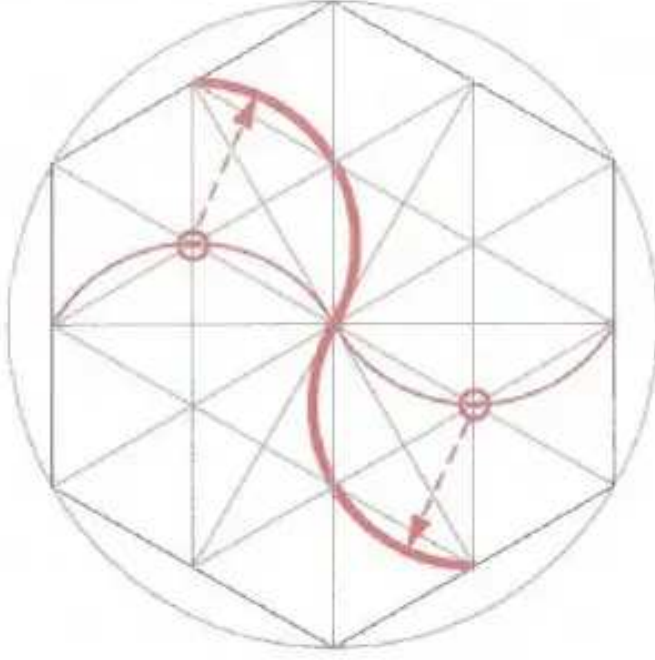
5 Pergelinizin ucunu ikinci bir çift yay oluşturmak için sırasıyla birinci ve ikinci yayın üst ve alt noktasında yer alan yuvarlak içine alınmış kesişim noktalarına yerleştirin.
