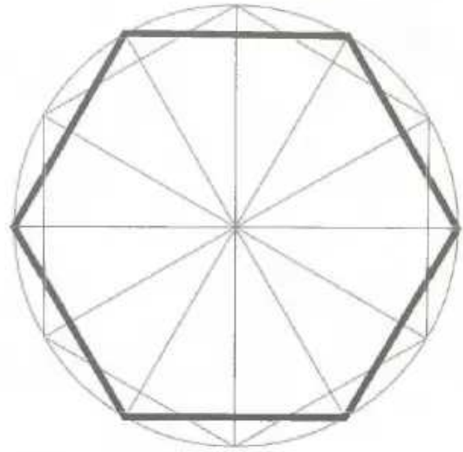
2 Dairenin içine, görüldüğü gibi tam olarak oturan ikinci bir altıgen çizin.
