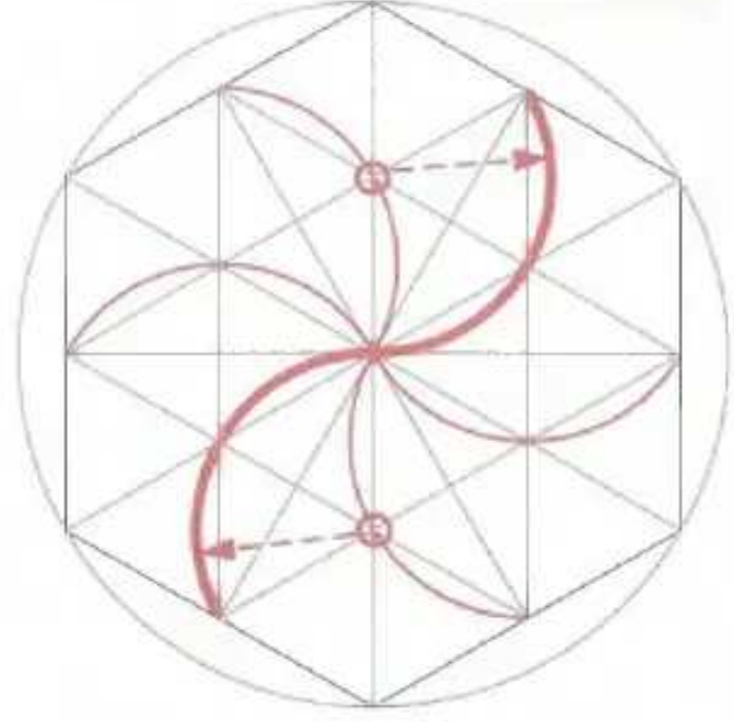
6 Pergelinizin ucunu yuvarlak içine alınmış kesişim noktalarına yerleştirerek üçüncü bir çift yay çizin. Bu altı yayın her biri merkezden kıvrılmaya başlayıp altıgenin farklı kenarlarına değmektedir.
