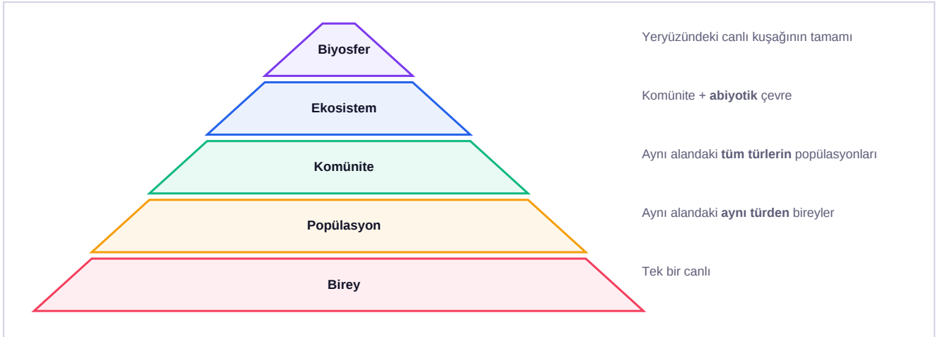
Şema 1 — Ekolojik organizasyon basamakları
