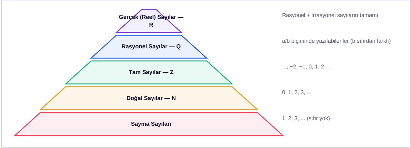
Şema 1 — Sayı kümelerinin iç içe yapısı
