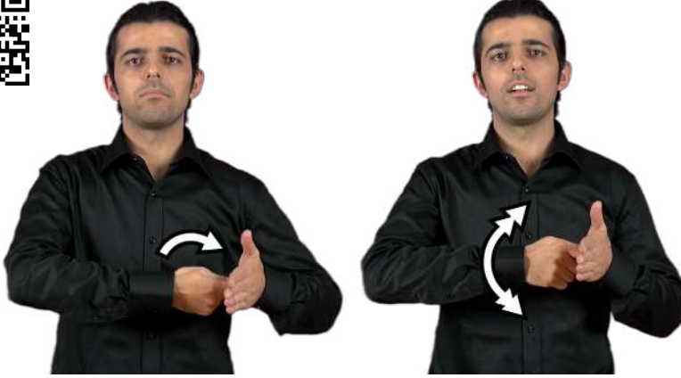
KİLITLEMEK
