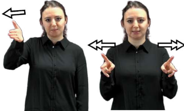
GİTMEK
