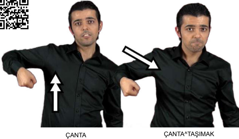
Şekil 4.61. TİD'de ÇANTA^TAŞIMAK.
