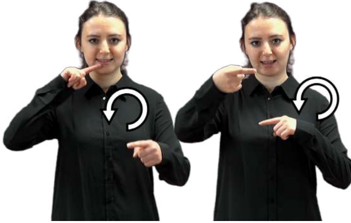
GELECEK^YIL
