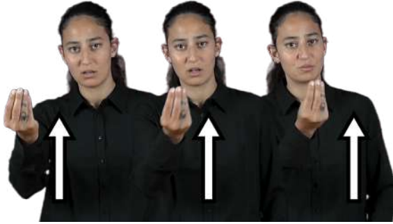
ÇIKMAK+yineleme/farklı konum.
