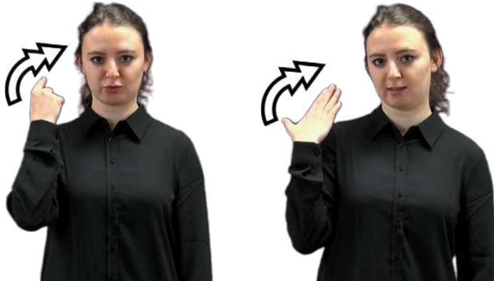
DÜN
