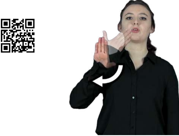
YOK
