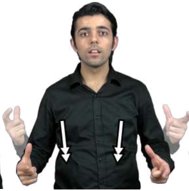
NEREDE
