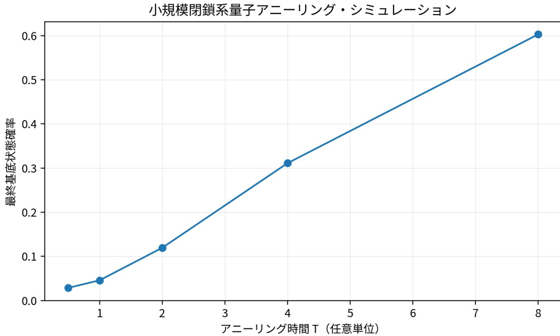
図 2: 小規模閉鎖系アニーリング・シミュレーションの最終基底状態確率
