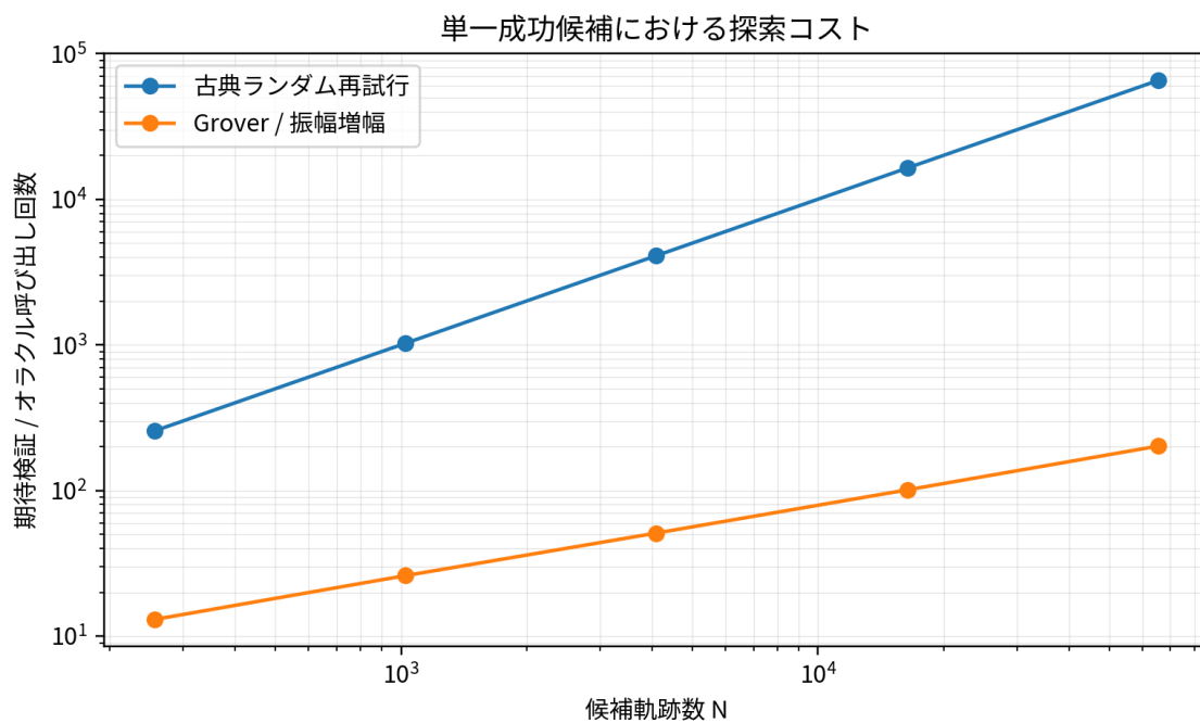
図 1: 単一成功候補における古典ランダム再試行と Grover/振幅増幅の期待検証・オラクル呼び出し回数
