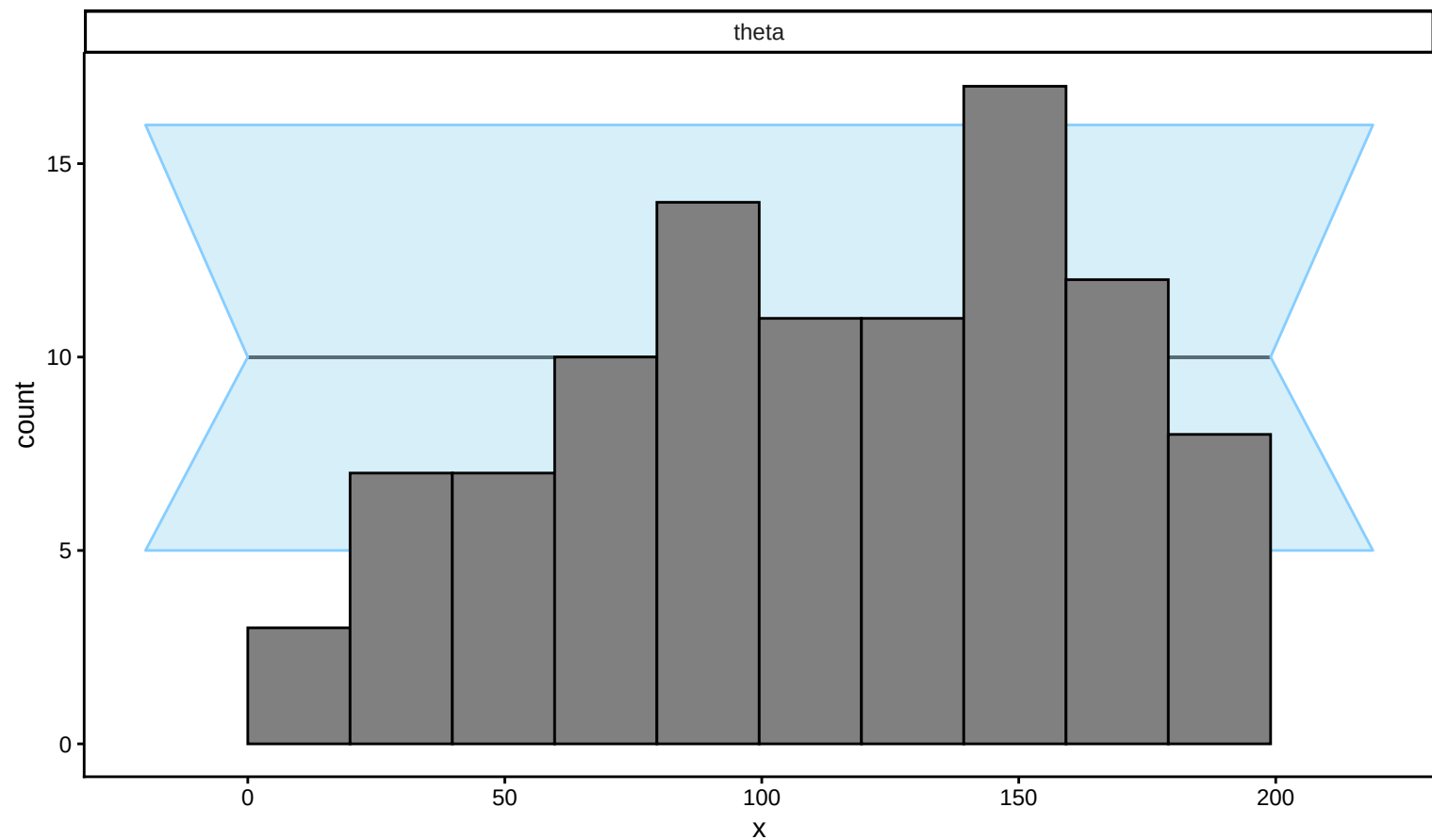
Posterior SBC: Simple Biased Agent
