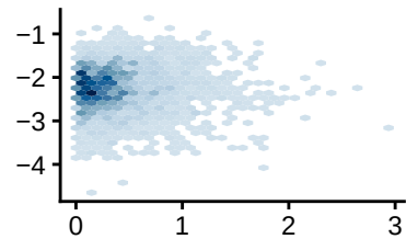
pop_log_q_sd
