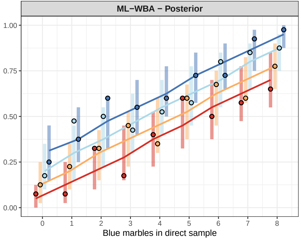
ML-WBA Posterior Population Posterior Predictive Check
