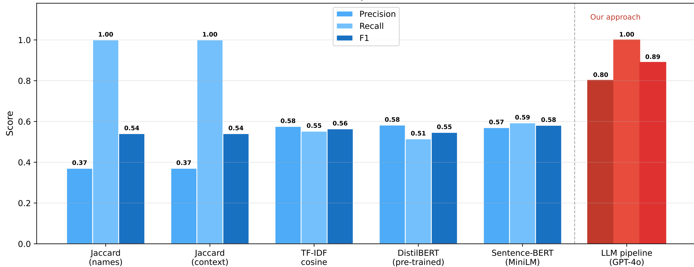
Baseline Methods vs. LLM Pipeline — Precision / Recall / F1
