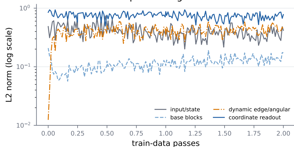
D Post-clip module gradient norms
