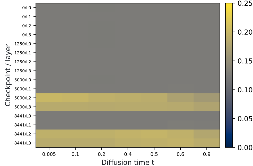
(d) Maximum slot mass
