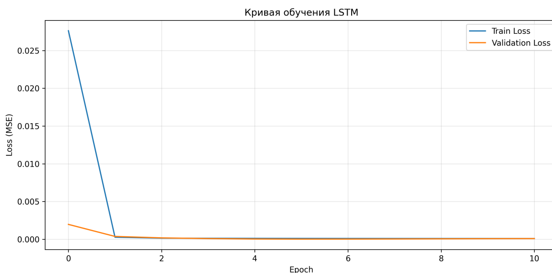
Рис. 3.4: Динамика функции потерь (MSE) в процессе обучения модели LSTM
