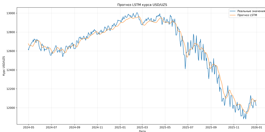
Рис. 3.5: Сравнение фактических и прогнозных значений курса USD/UZS (модель LSTM)
