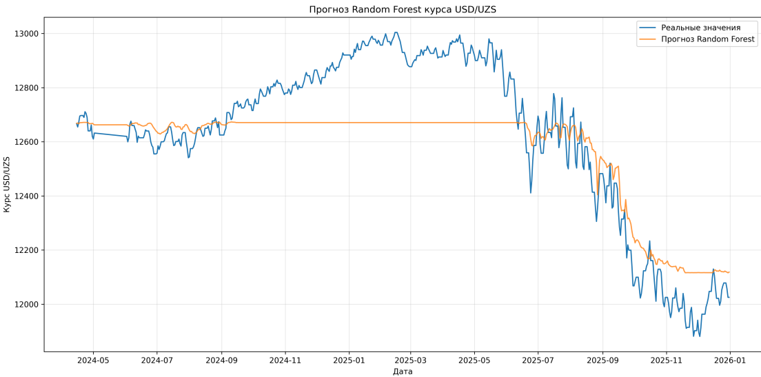
Рис. 3.2: Сравнение реальных и прогнозируемых значений модели Random Forest(30 лагов)
