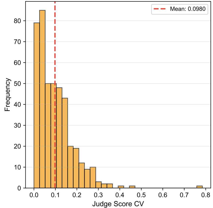
(D) Judge Score Dispersion
