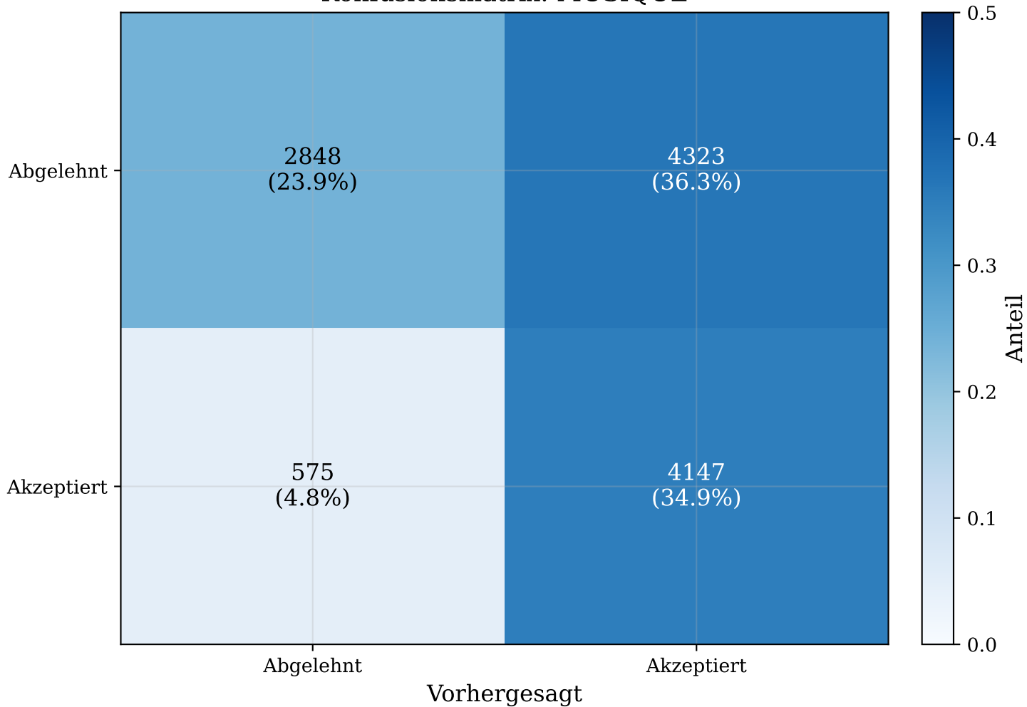
Konfusionsmatrix: MUSIQUE
