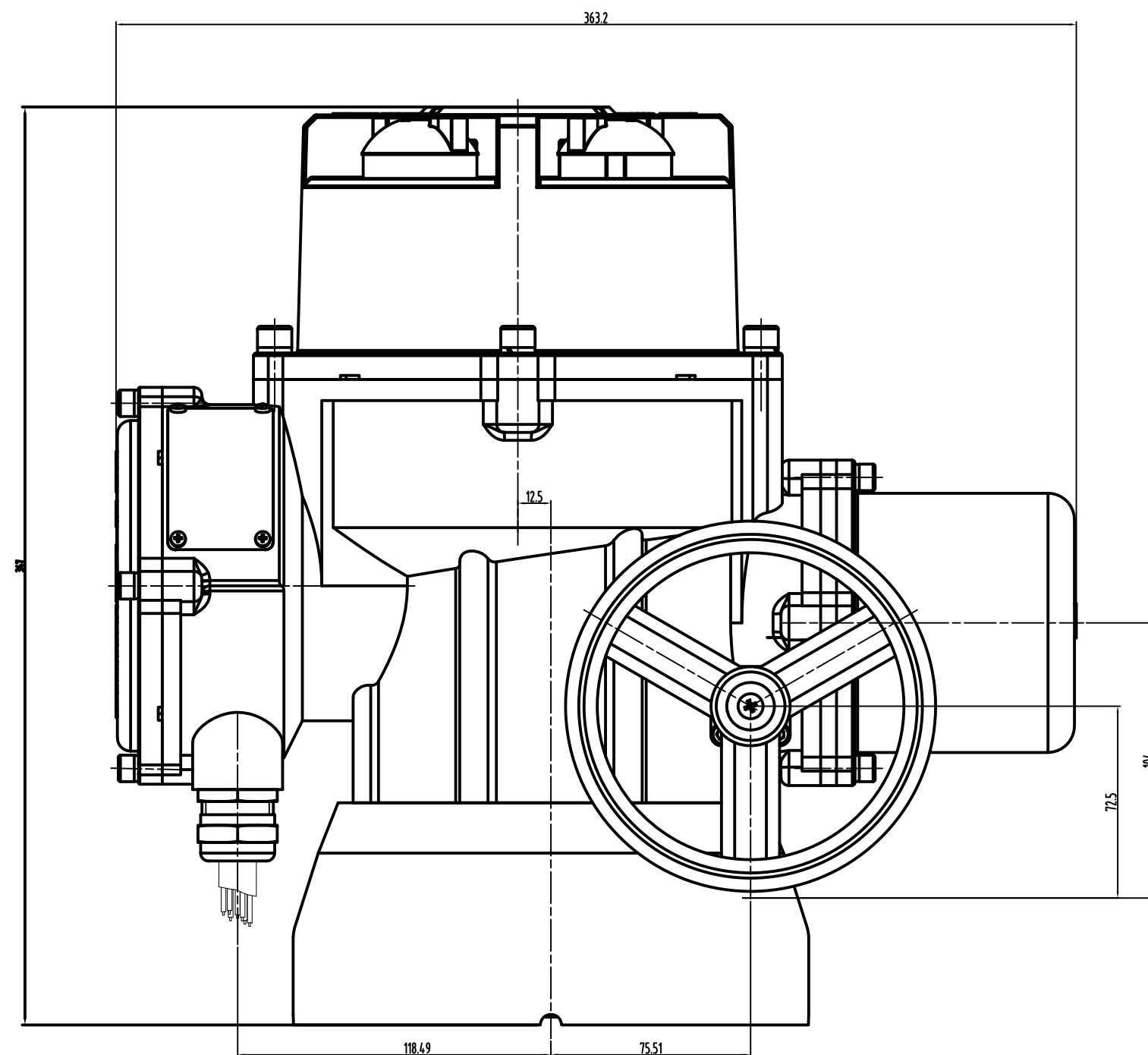
RL80~100外型图
