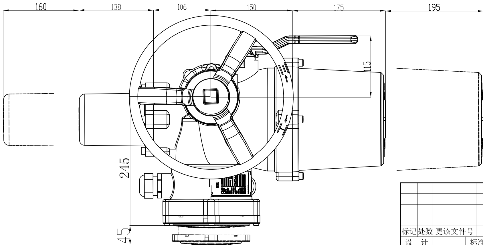
RQML06直行程外型图
