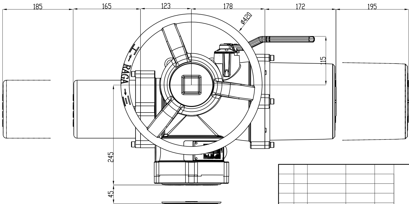
RQML54直行程外型图
