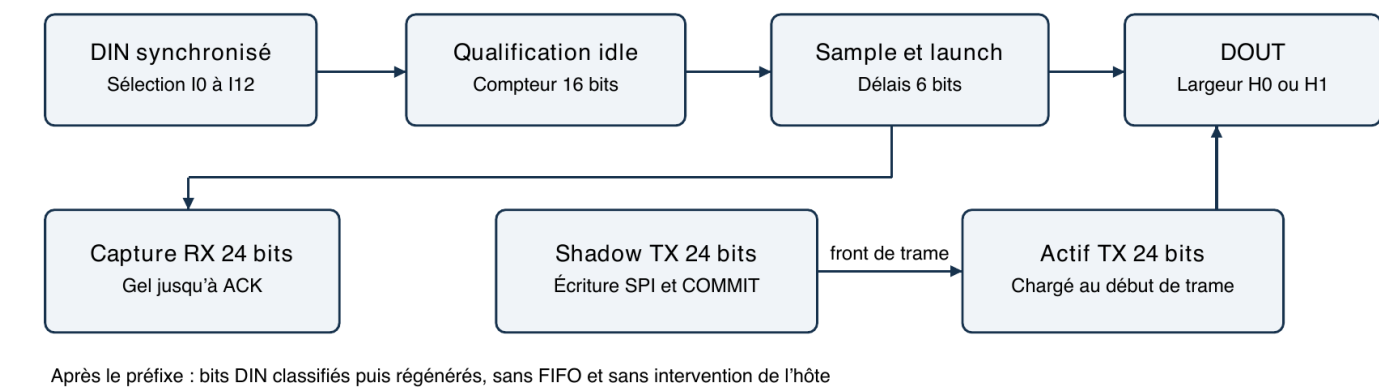
Figure 3 Chemin de données du moteur temporel
