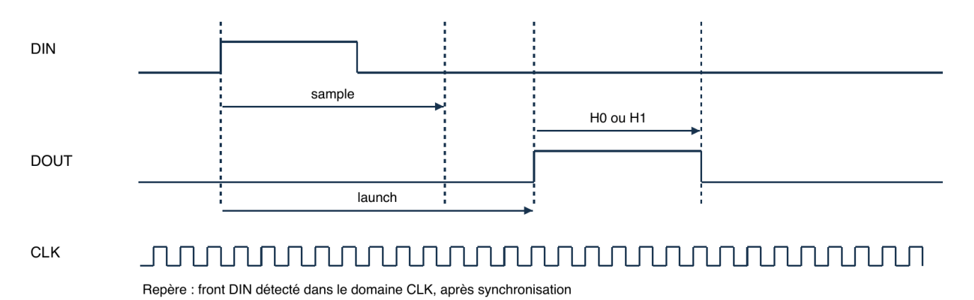
Figure 4 Chronogramme de principe ; non   l chelle
