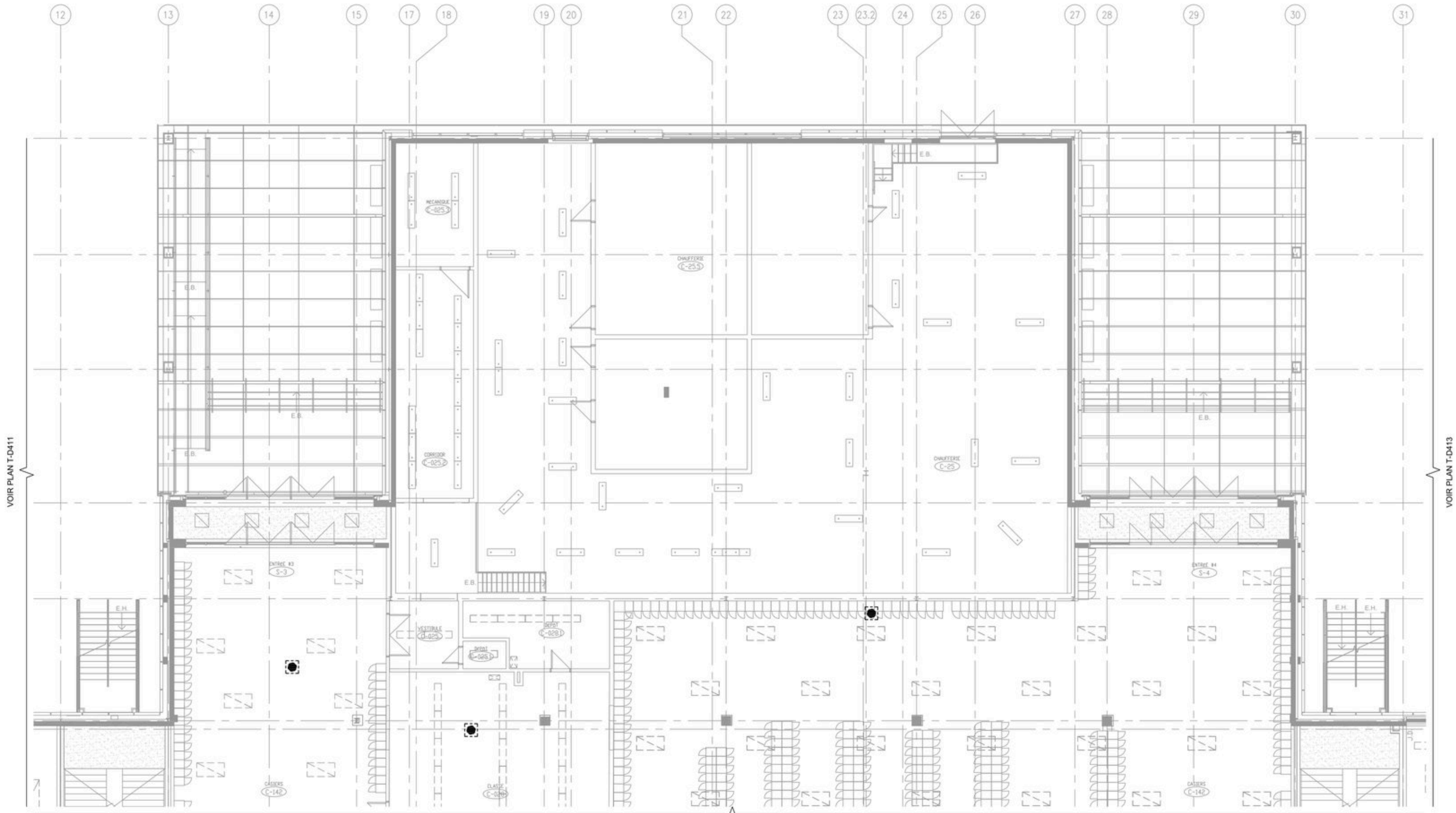
01 REZ-DE-CHAUSSEE - BLOC C1 - EXISTANT/ DÉMOLITION T-D412/ ÉCHELLE : 1:100
