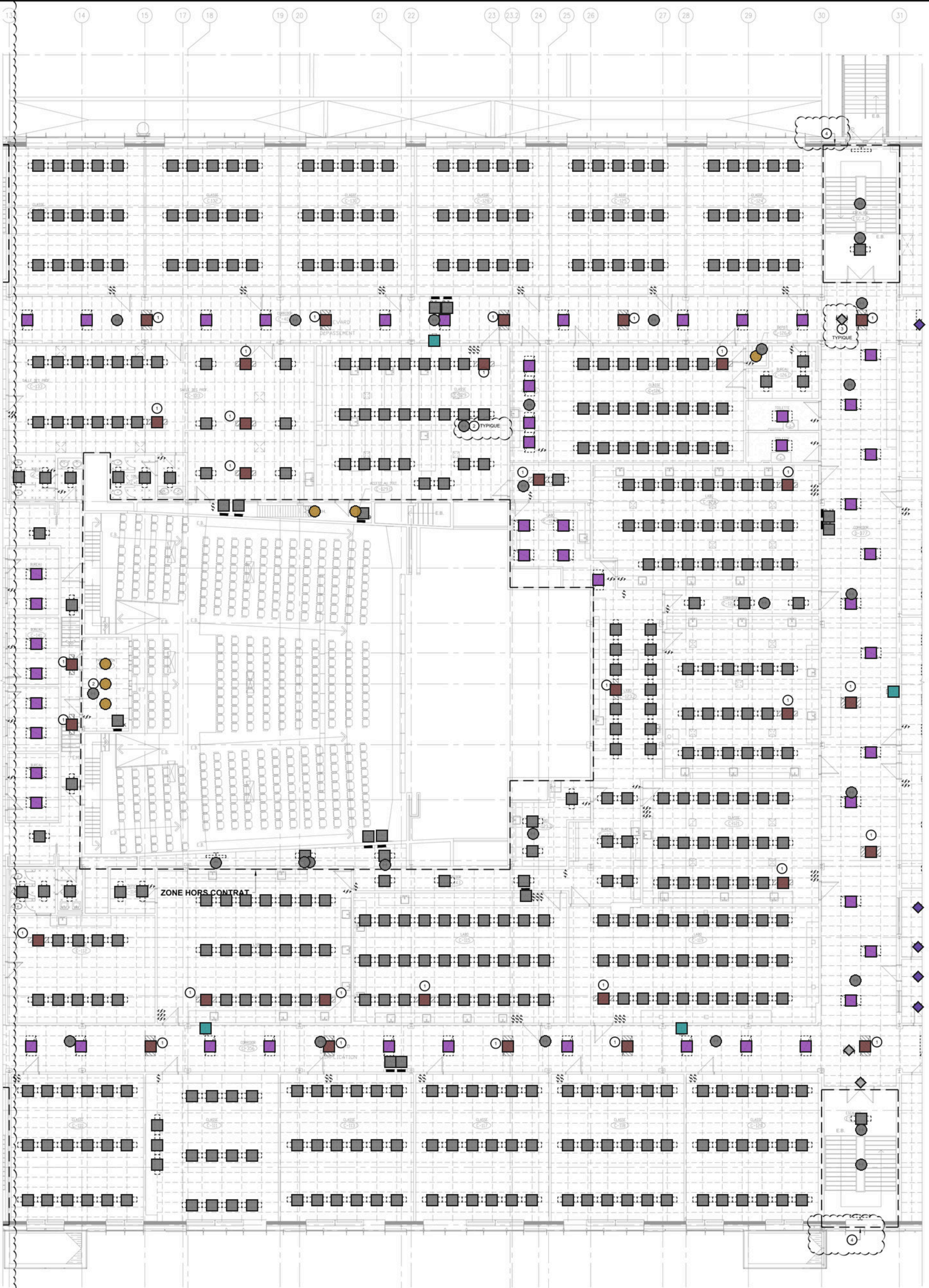
01 ÉTAGE - BLOC C - EXISTANT/ DÉMOLITION E-D221 ÉCHELLE: 1/100
