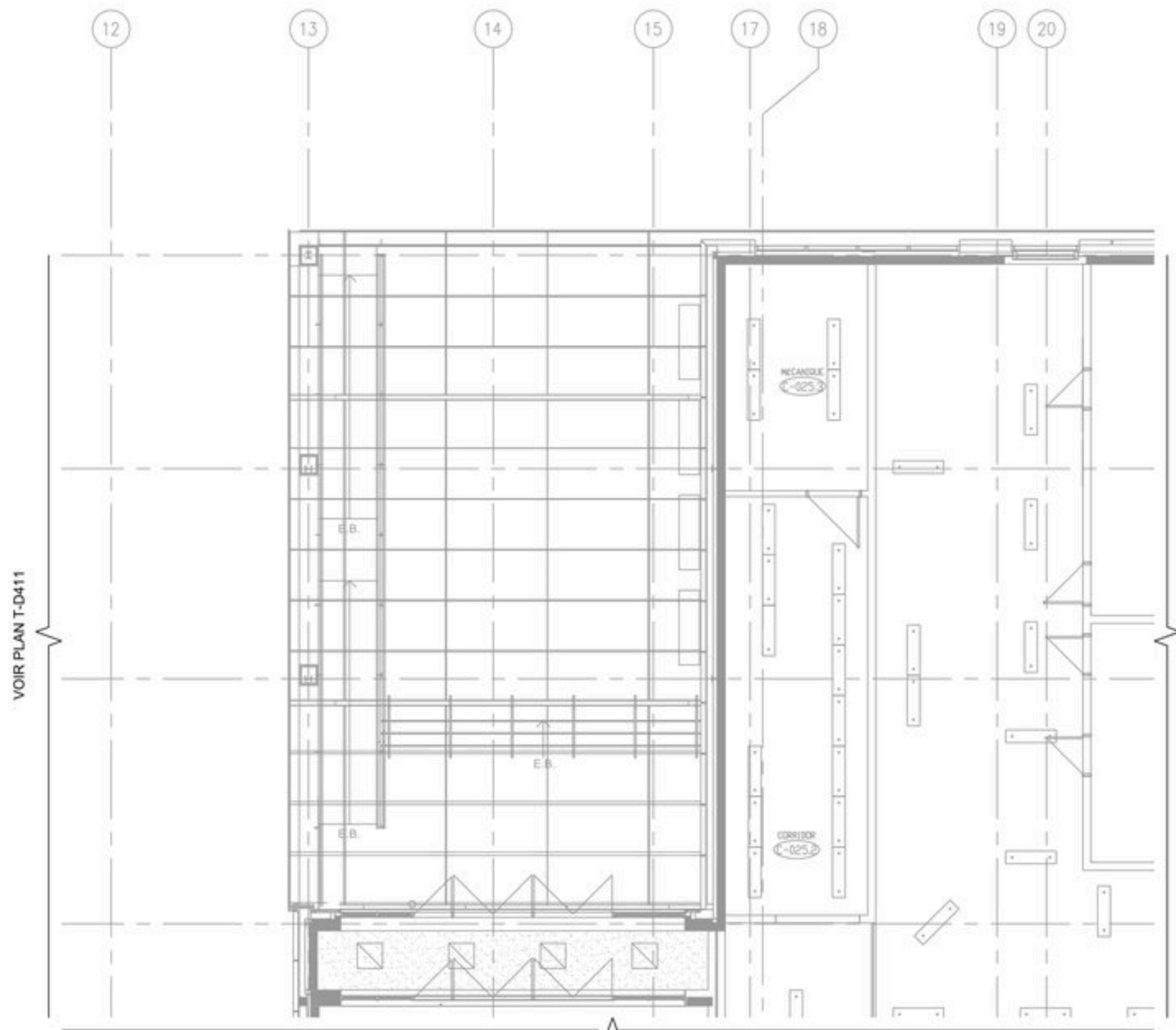
01 EXTRAIT SALLE ÉLECTRIQUE - REZ-DE-CHAUSSEE - BLOC C1 - EXISTANT/ DÉMOLITION T-D412/ ÉCHELLE : 1:100
