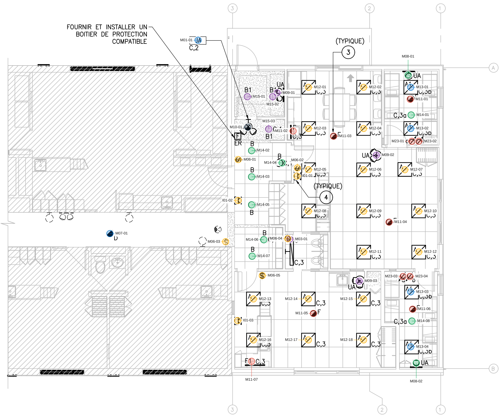
AMÉNAGEMENT - ÉCLAIRAGE ET ALARME INCENDIE ÉCHELLE 1/8" = 1'-0"
