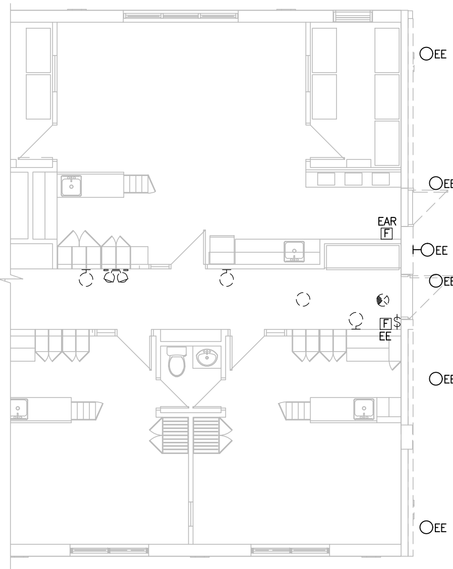
DÉMANTÈLEMENT - ÉCLAIRAGE ET ALARME INCENDIE ÉCHELLE 1/8" = 1'-0"
