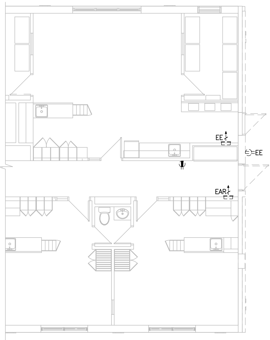
DÉMANTÈLEMENT - SERVICES ÉCHELLE 1/8" = 1'-0"
