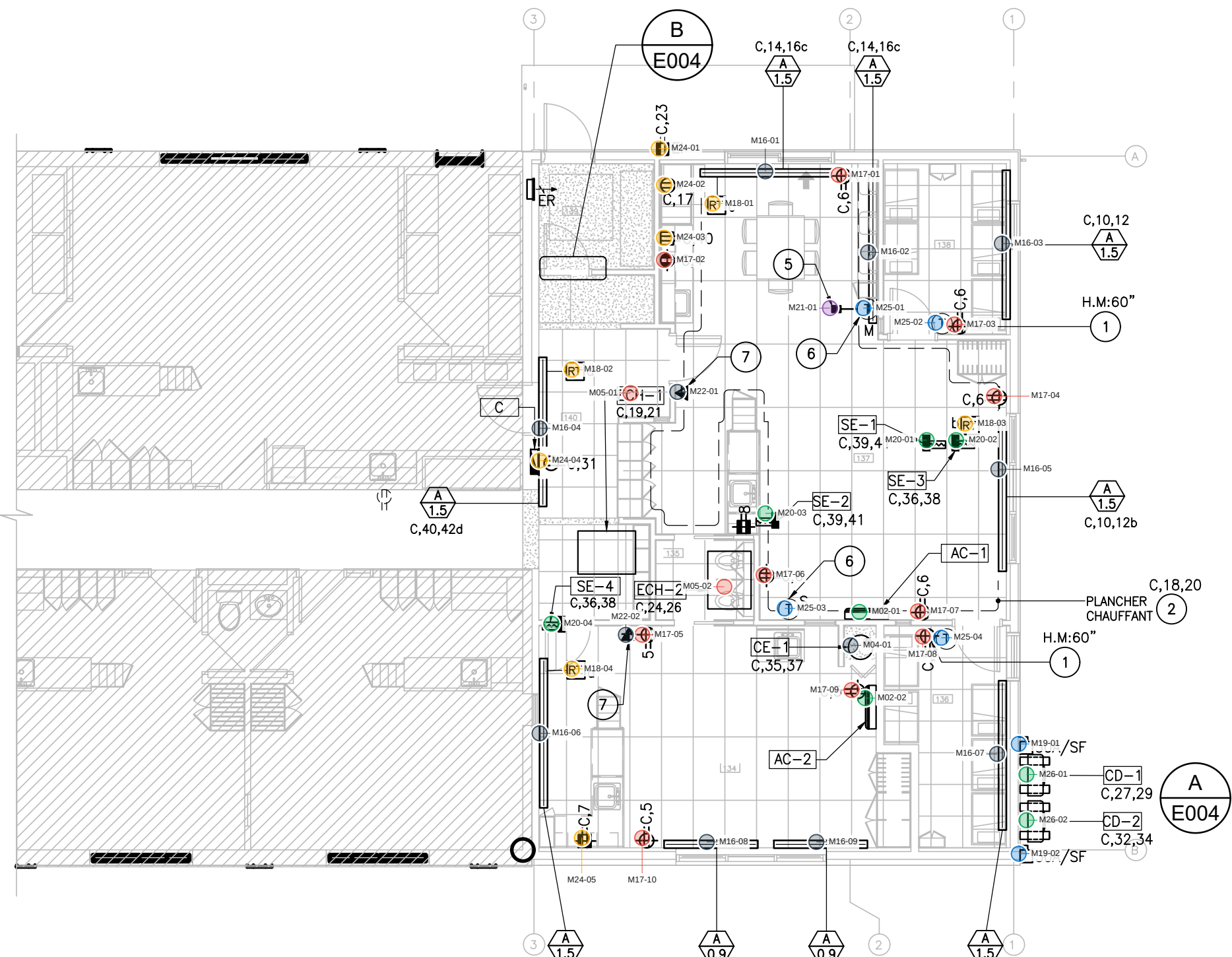
AMÉNAGEMENT - SERVICES ÉCHELLE 1/8" = 1'-0"
