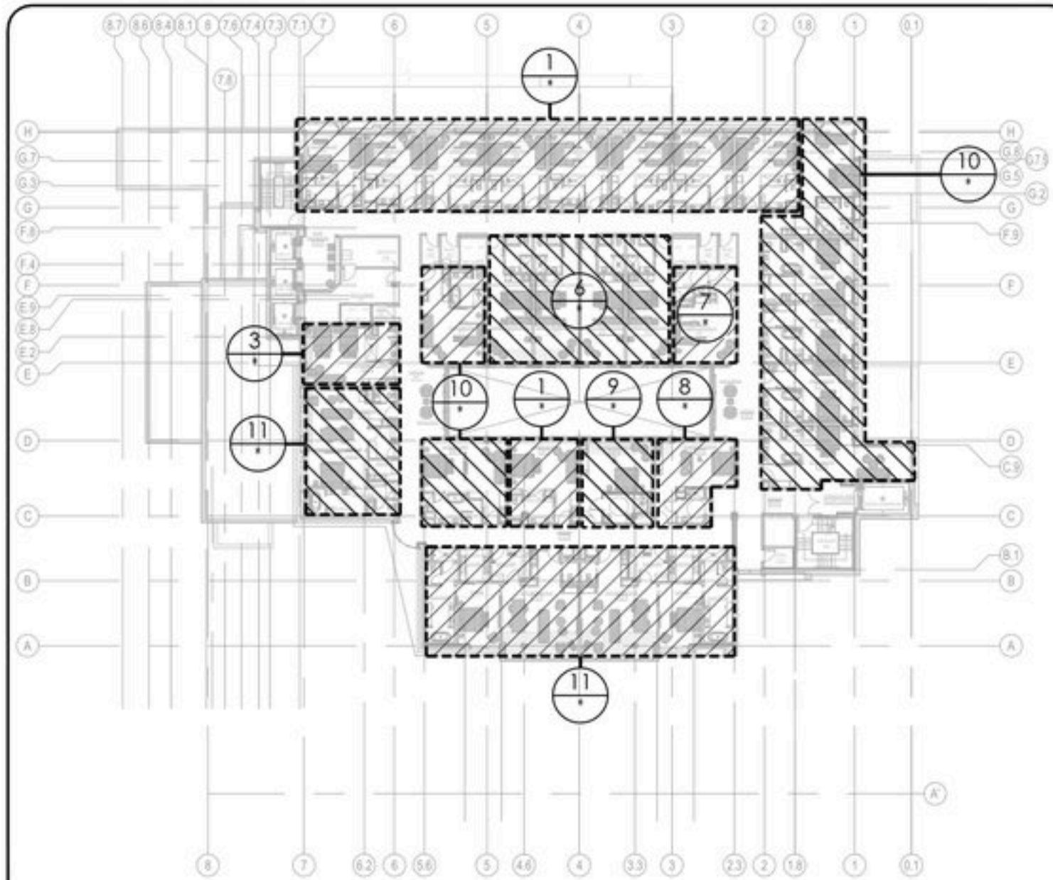
PLAN CLÉ - NIVEAU 6 ÉCHELLE : 1/32" = 1'-0"
