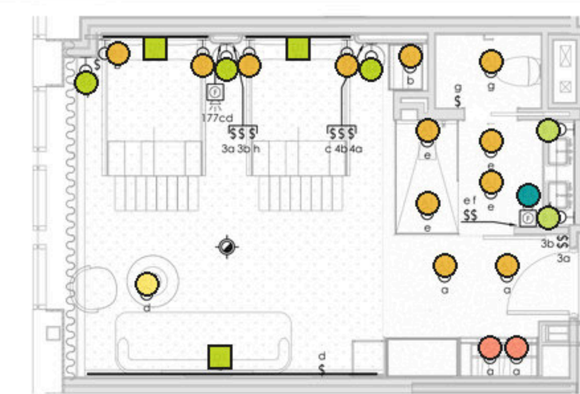
CHAMBRE DOUBLE 1 ÉCHELLE : 1/4" = 1'-0"
