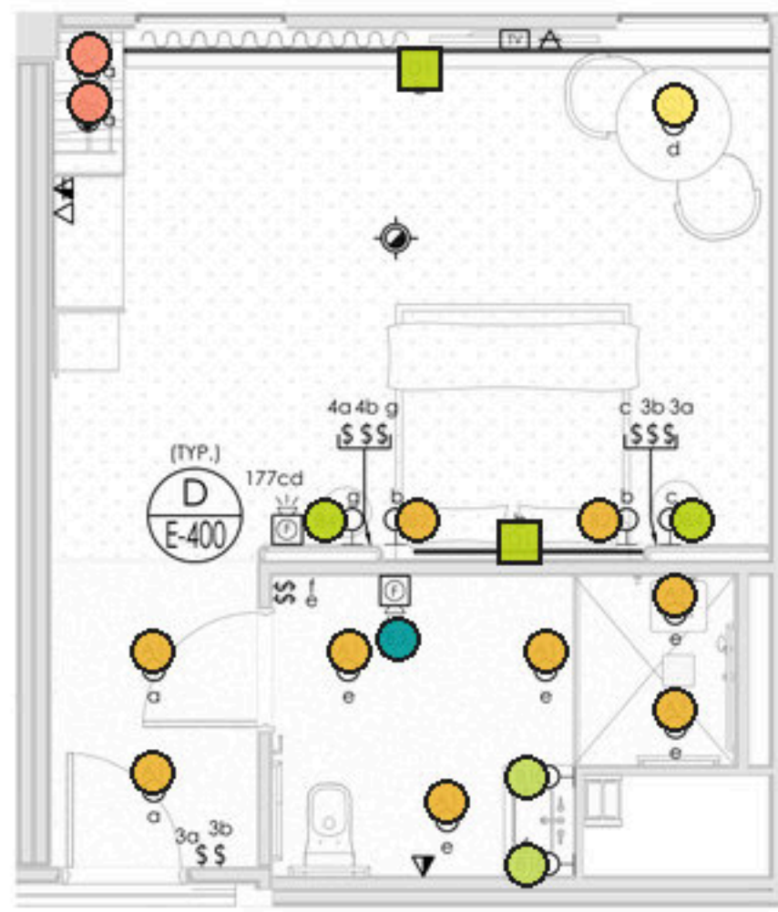
CHAMBRE UNIVERSELLE 3 ÉCHELLE : 1/4" = 1'-0"
