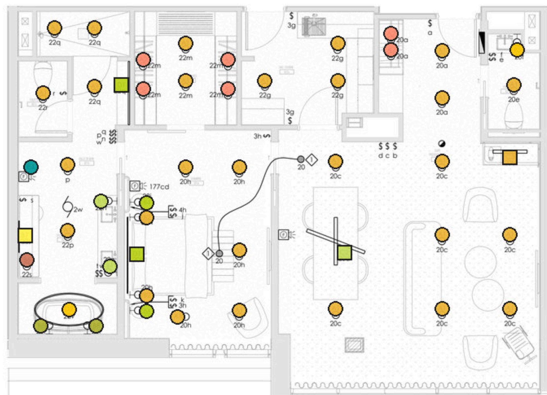
SUITE PRÉSIDENTIELLE ÉCHELLE : 1/4" = 1'-0"
