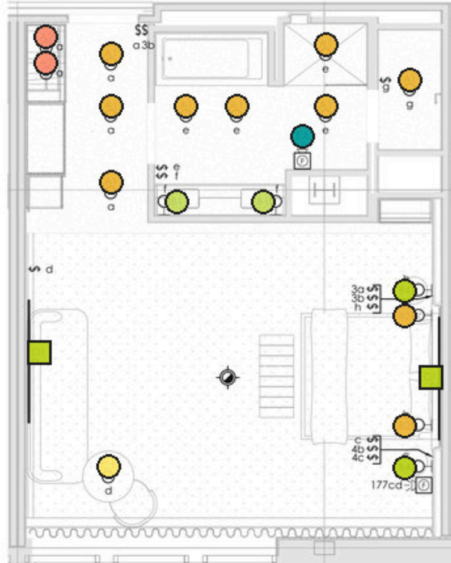
SUITE PRESTIGE 1 ÉCHELLE : 1/4" = 1'-0"
