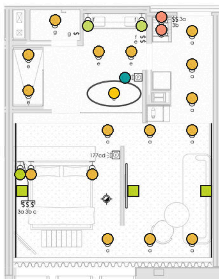
SUITE PRESTIGE 2 (523) ÉCHELLE : 1/4" = 1'-0"
