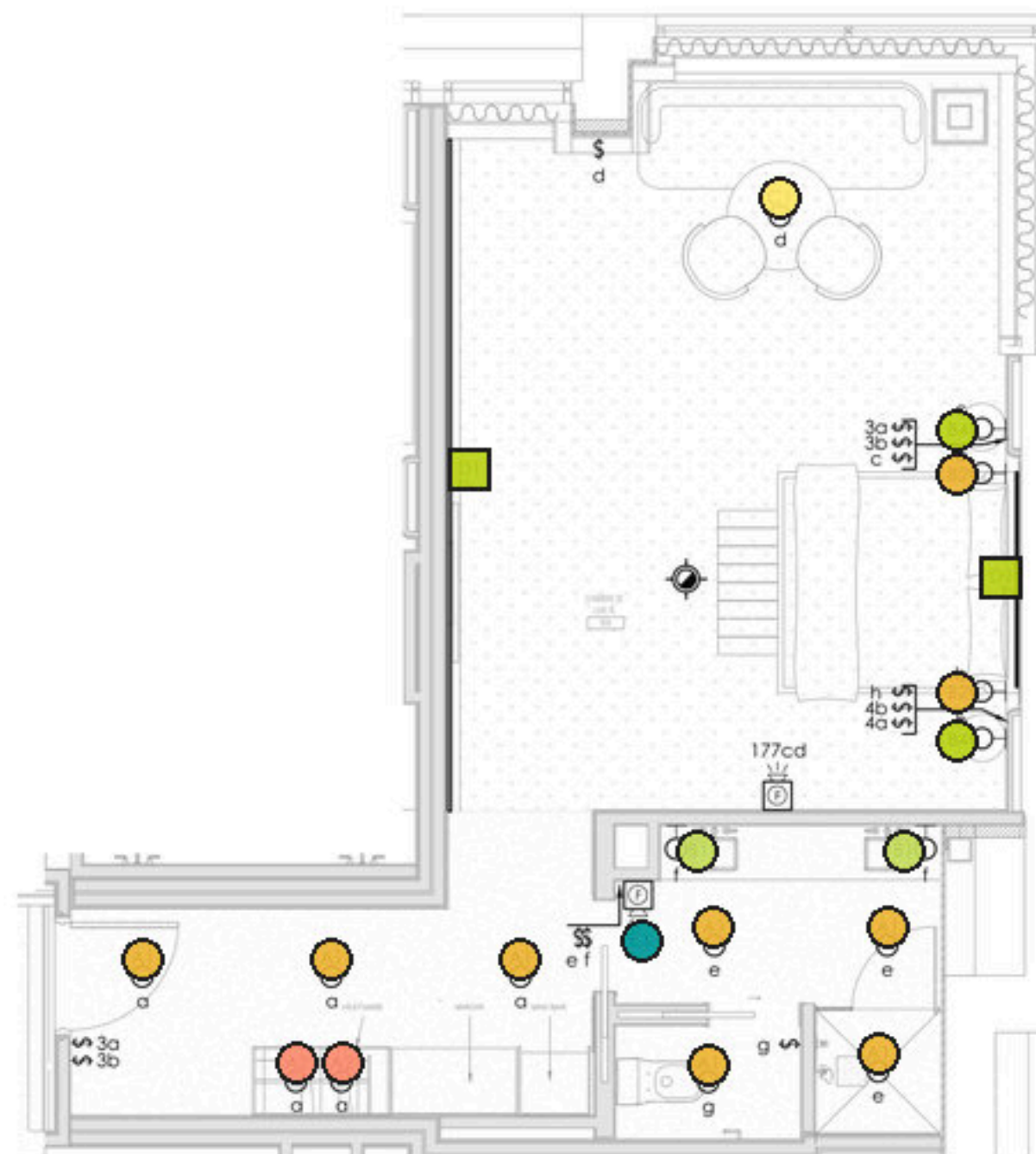
CHAMBRE DE LUXE XL ÉCHELLE : 1/4" = 1'-0"
