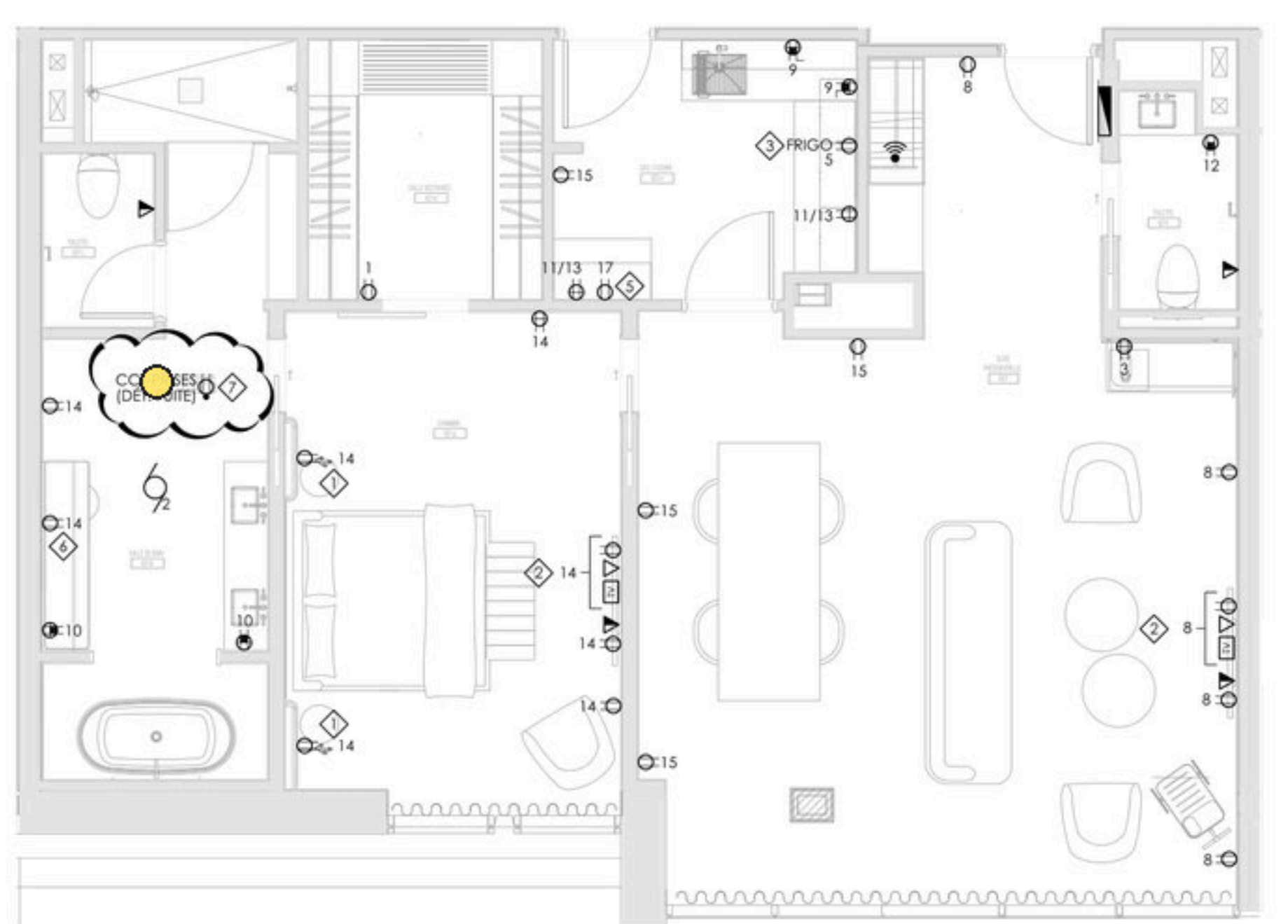
SUITE PRÉSIDENTIELLE 11 ÉCHELLE : 1/4" = 1'-0"
