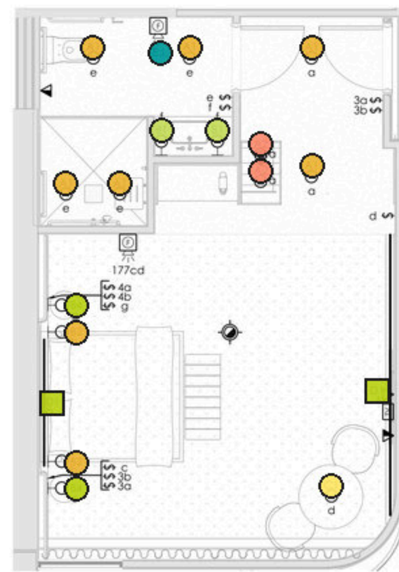
CHAMBRE UNIVERSELLE 1 ÉCHELLE : 1/4" = 1'-0"
