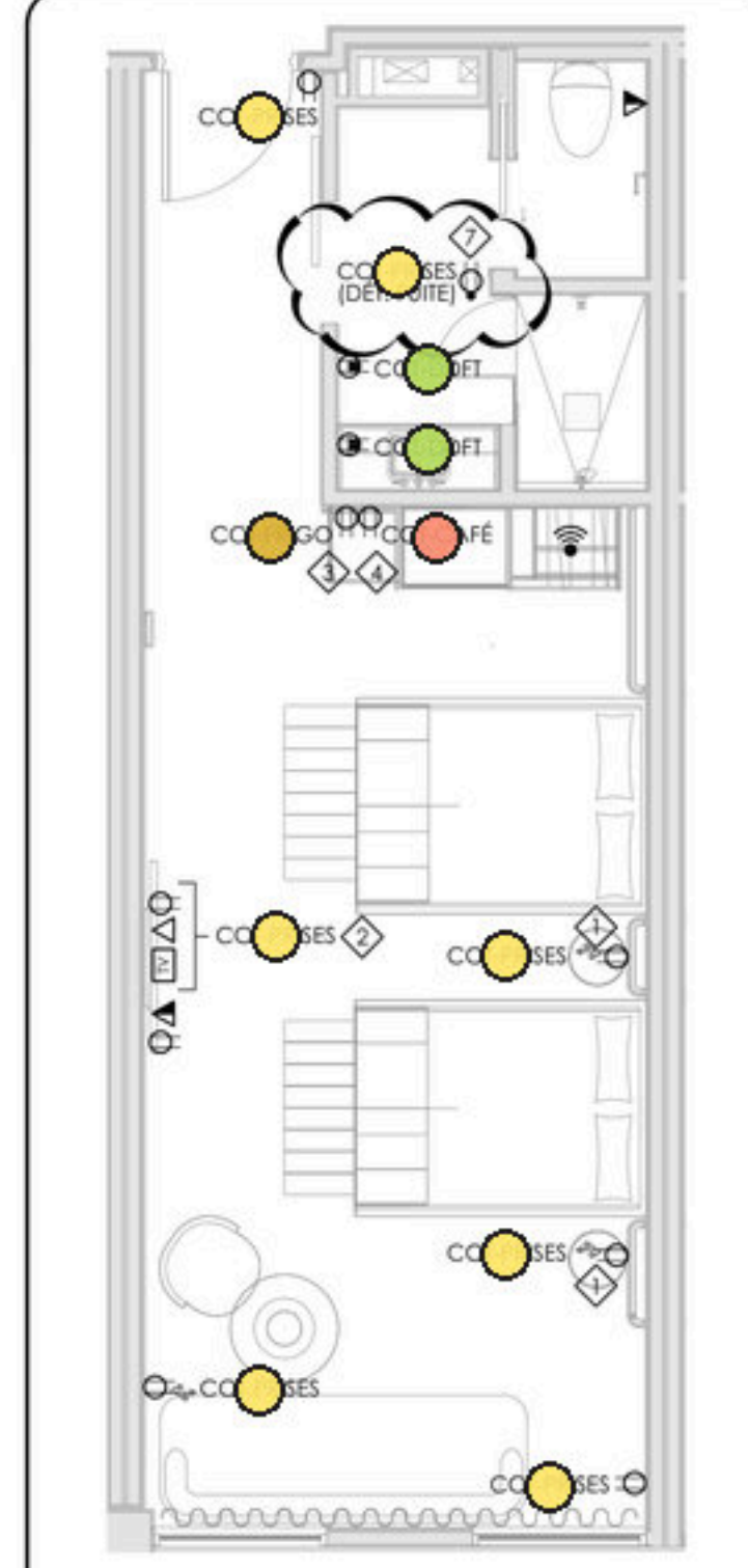
CHAMBRE DOUBLE 2 6 ÉCHELLE : 1/4" = 1'-0"
