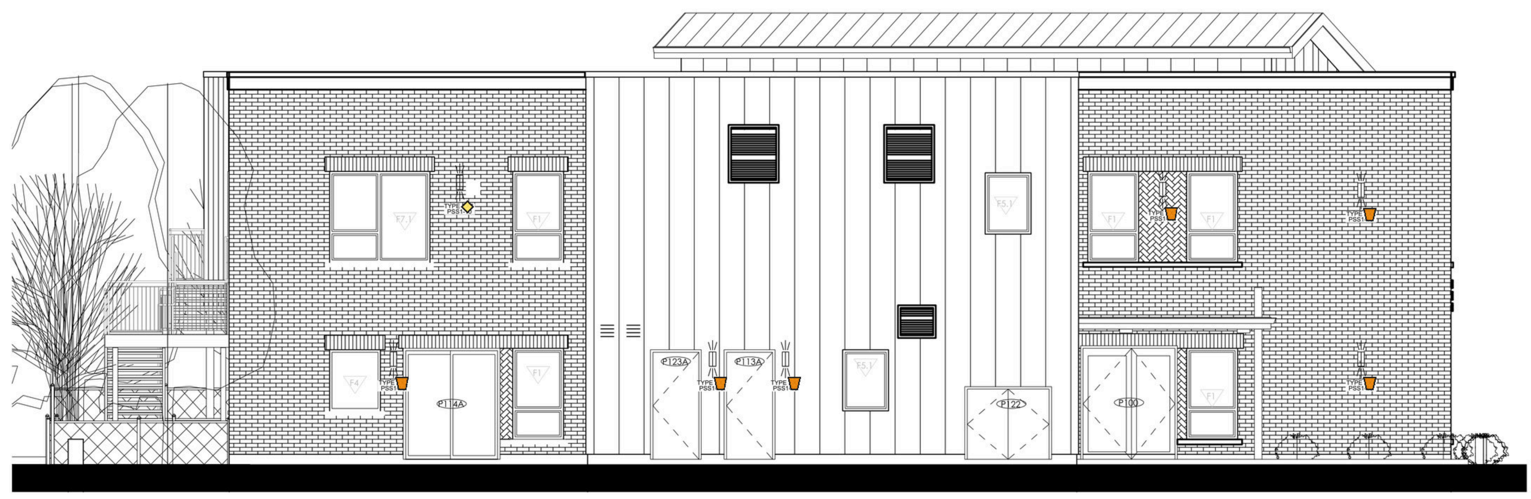
2 ÉLEVATION LATÉRALE OUEST- STATIONNEMENT VOISIN E-051 1 : 50
