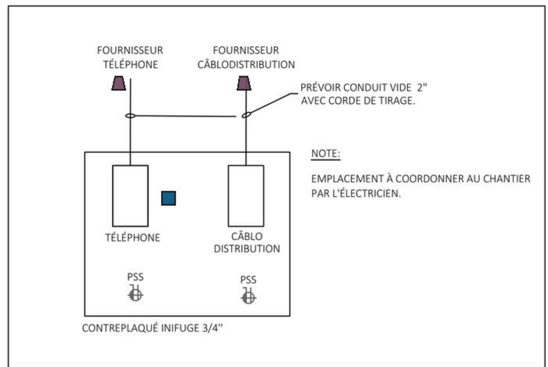
INSTALLATION TYPIQUE CONTREPLAQUÉ CABLODISTRIBUTION ÉCHELLE: AUCUNE
