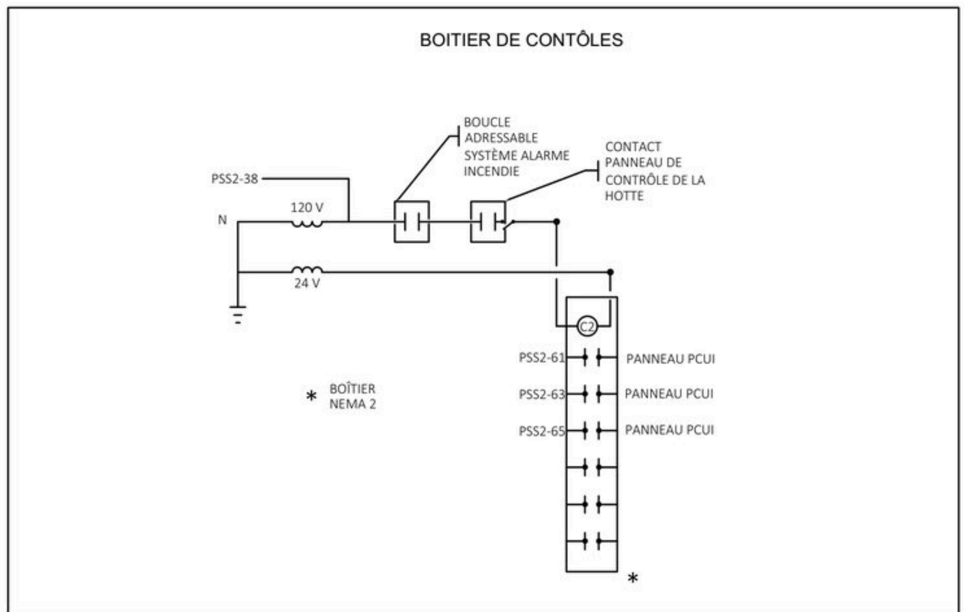
CONTACTEUR POUR CUISINE - C2 ÉCHELLE: AUCUNE
