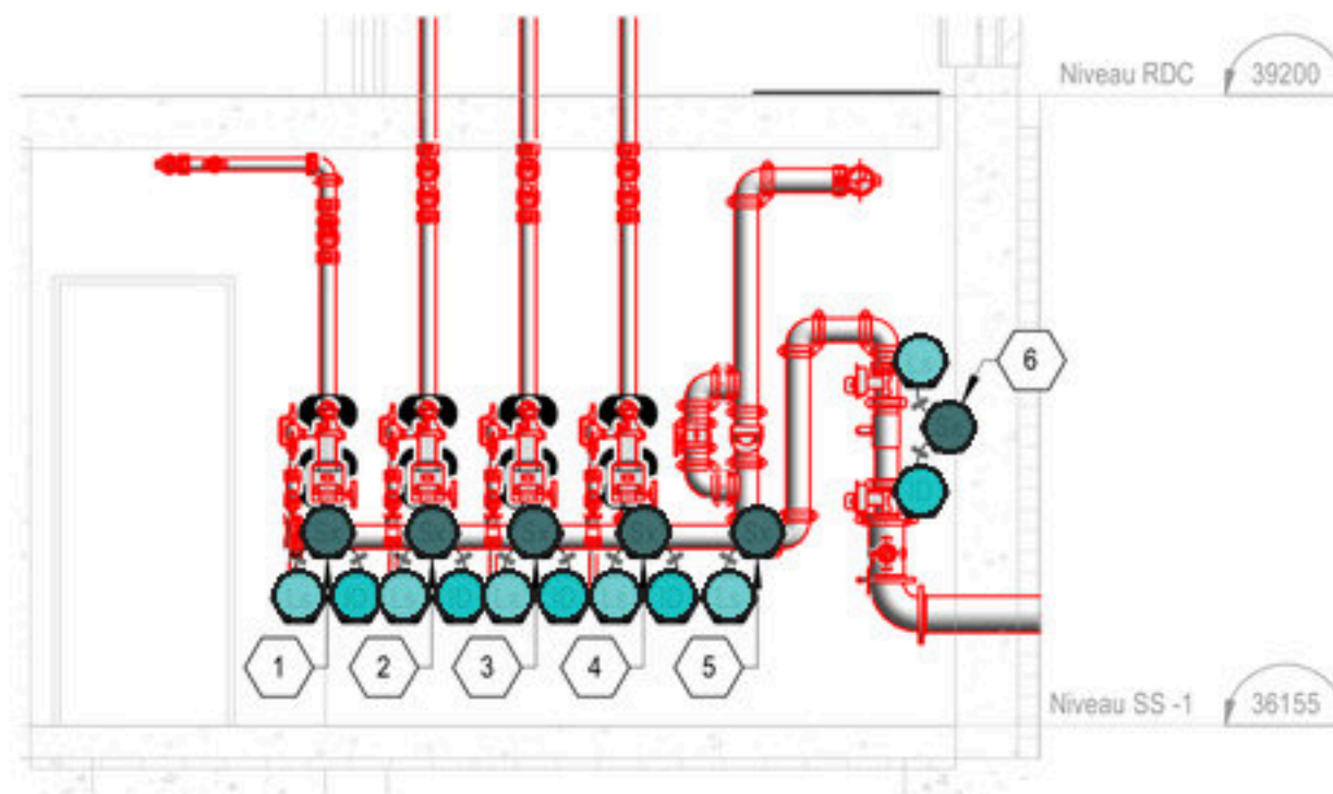
ENTRÉE D'EAU Echelle: N.A.E.
