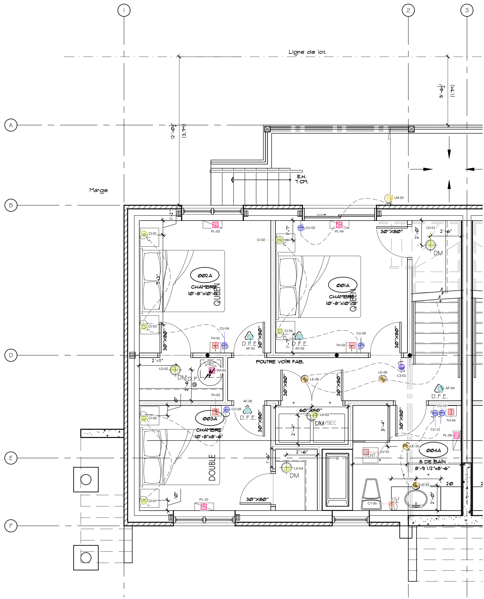
UNITÉ TYPE A - PLAN SOUS-SOL NOUVELLE CONDITION ÉCHELLE 1/4"=1'-0" A-801
