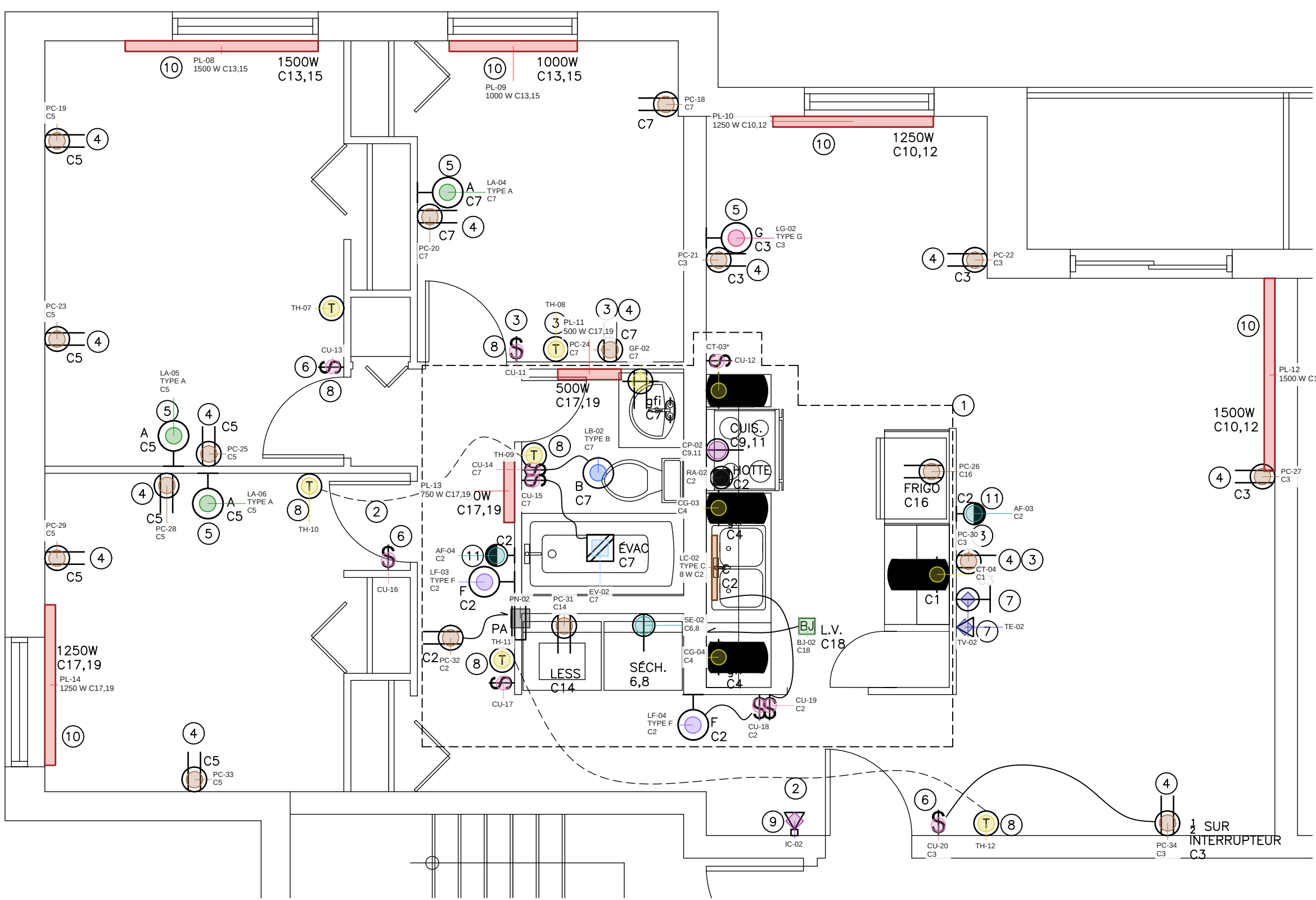
LOGEMENT TYPE B (3E ÉTAGE)
