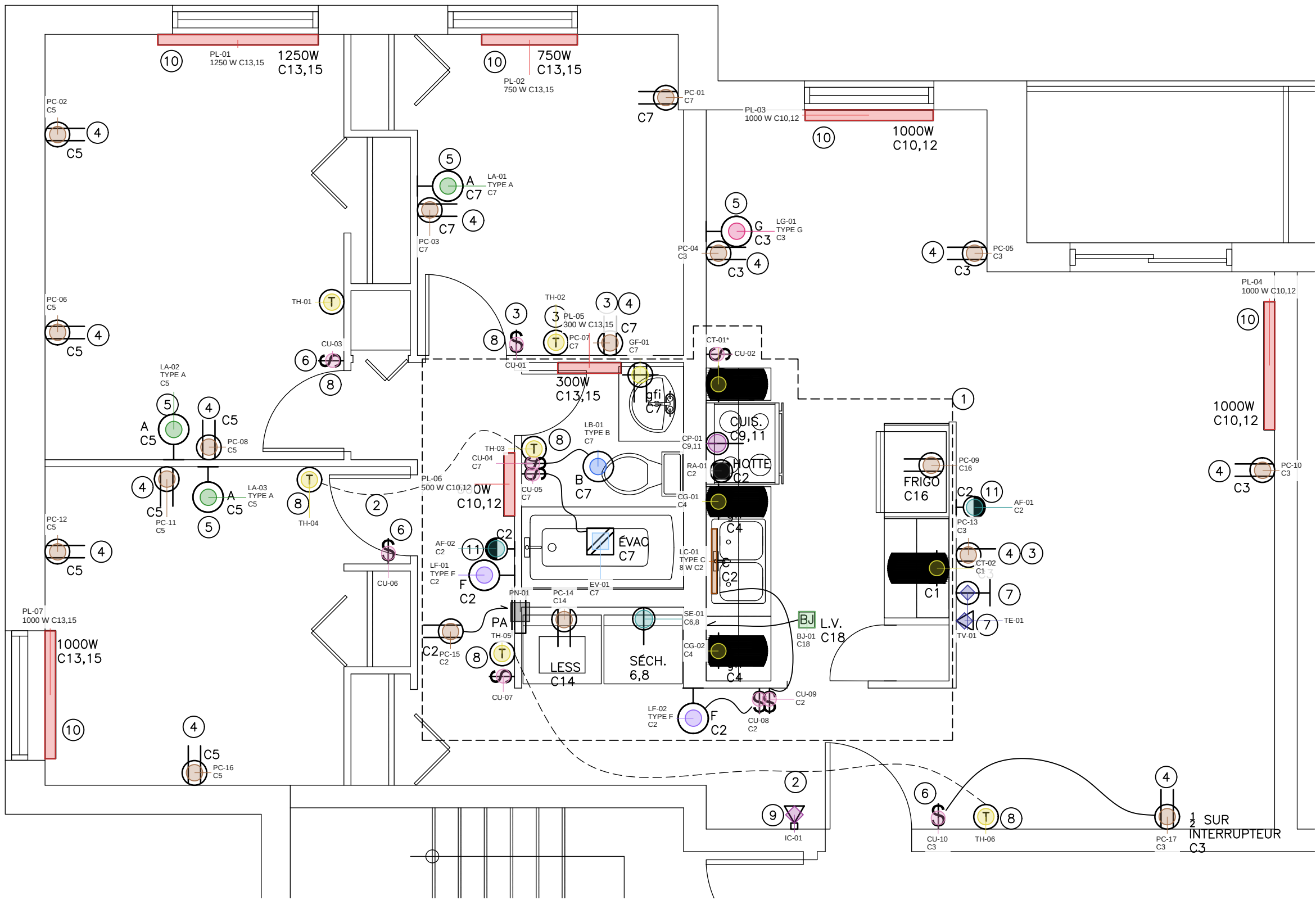
LOGEMENT TYPE A (RDC ET 2E ÉTAGE)
