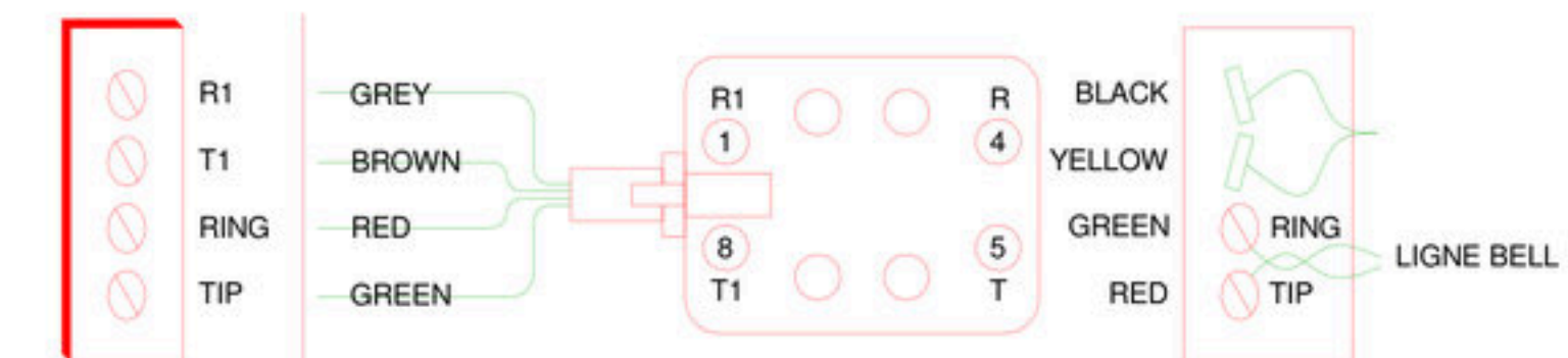
DÉTAIL DE RACCORDEMENT DU MODULE CA38A 1:1
