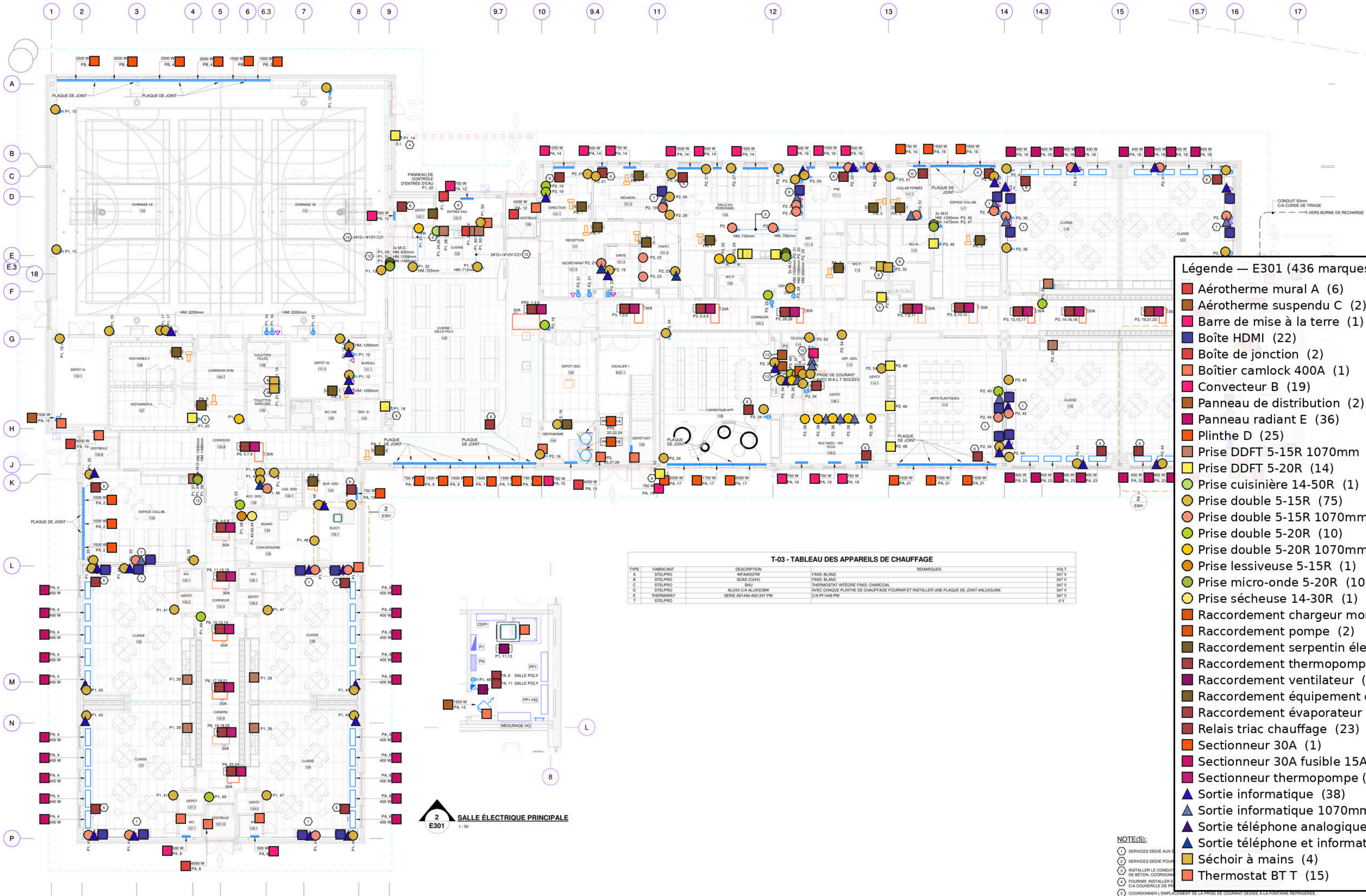
NIVEAU 1 - SERVICES 1:100
